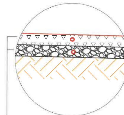
Detaliu C sc. 1:20
