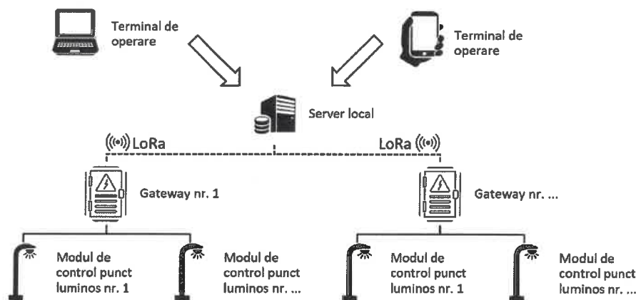
(Schema principiu de funcționare)
