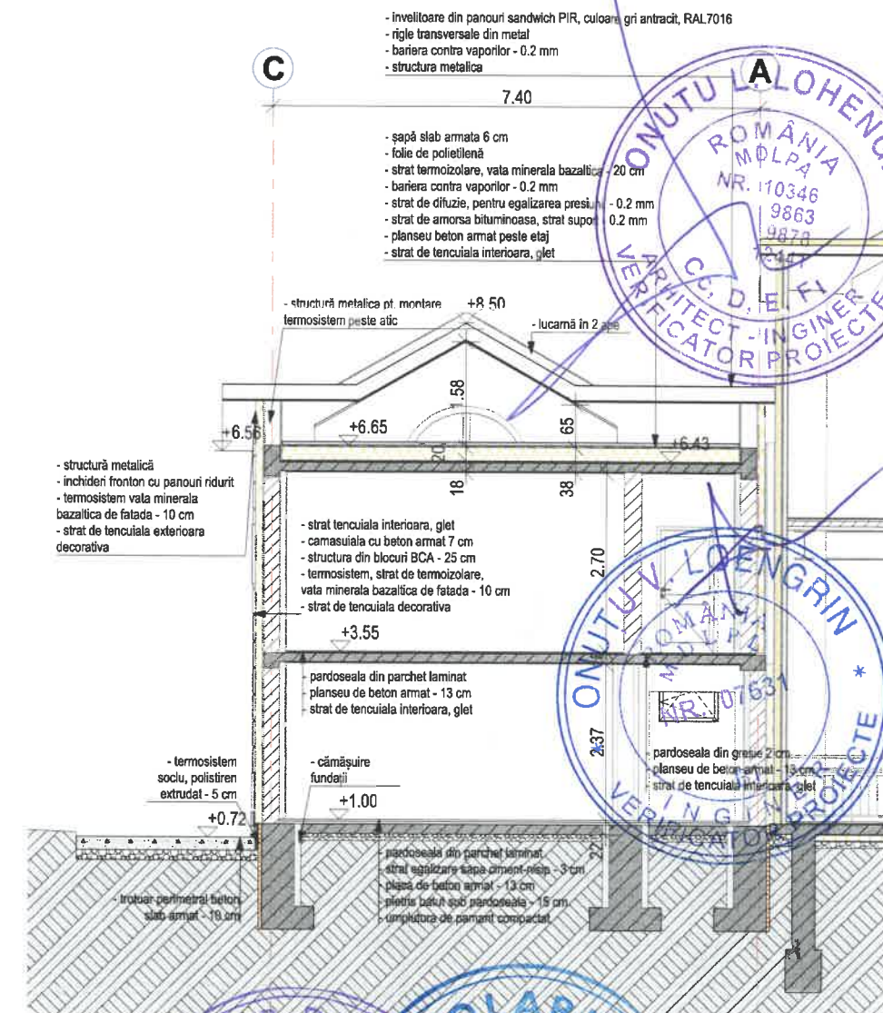
A SECTIUNE TRANSVERSALĂ
