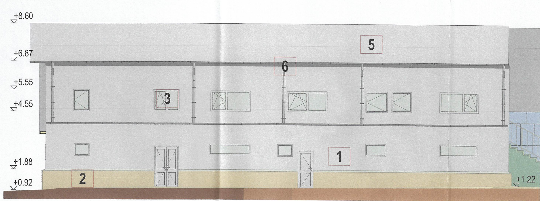
FATADA PRINCIPALA (LA STRADA)
