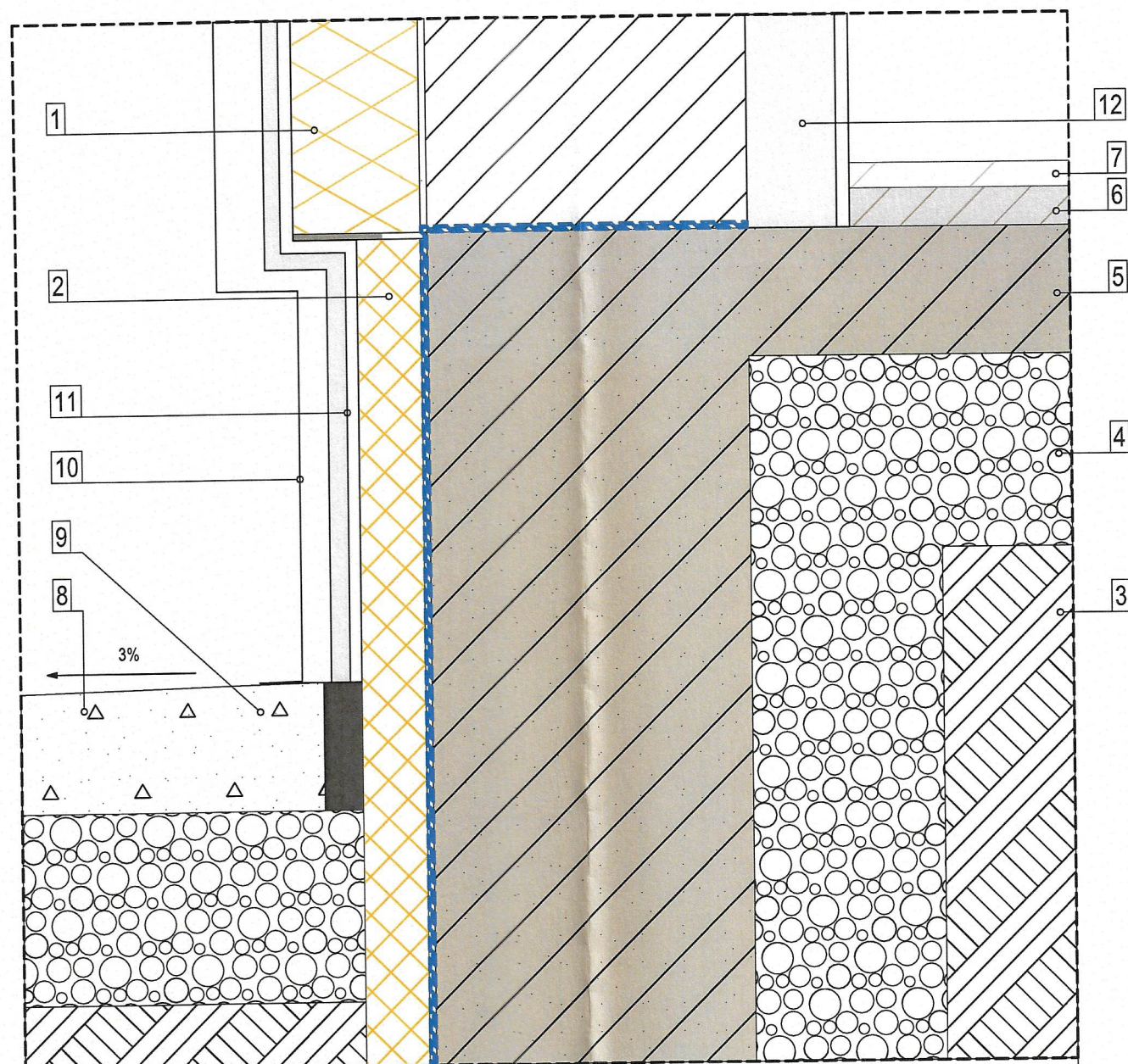
DETALIU SOCLU + PLACA PE SOL + TROTUAR
