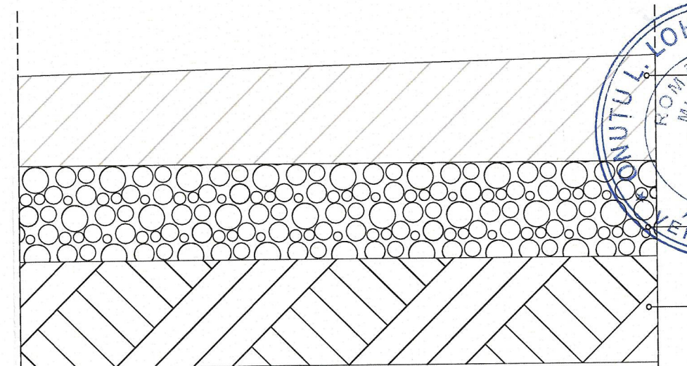
TROTUAR BETON ARMAT
