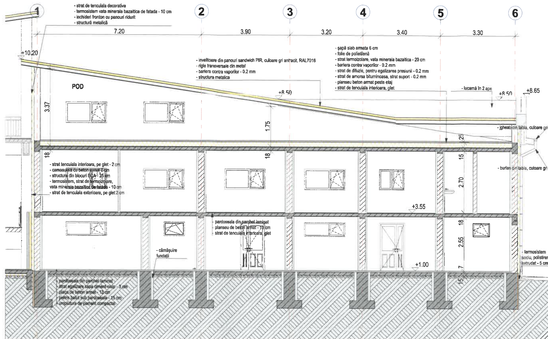
B SECTIUNE LONGITUDINALĂ
