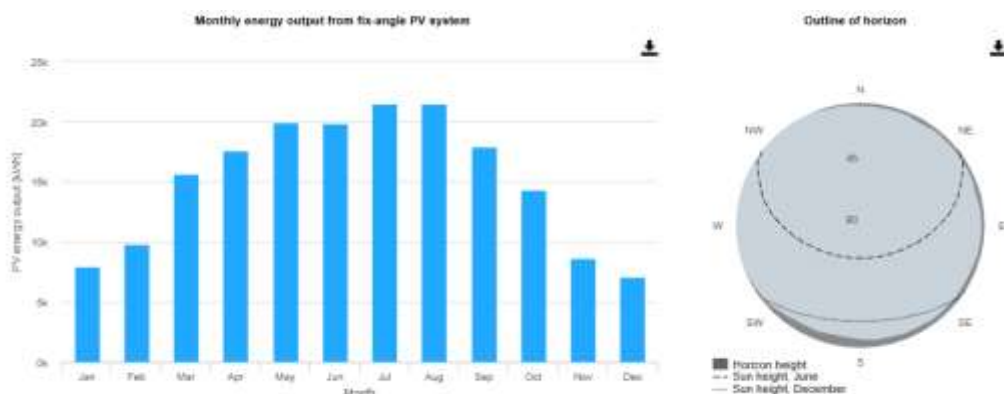
(Graficul de productie)
