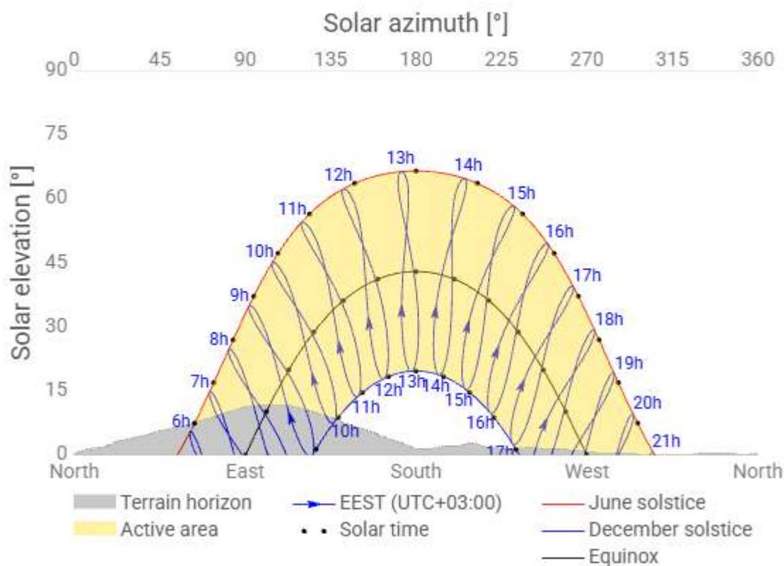
(Diagrama elevatie-azimut)
