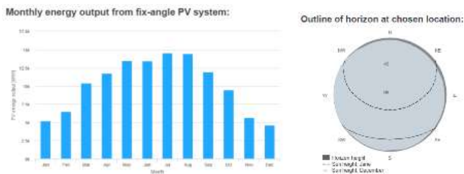
CF 71171(Graficul de productie)
