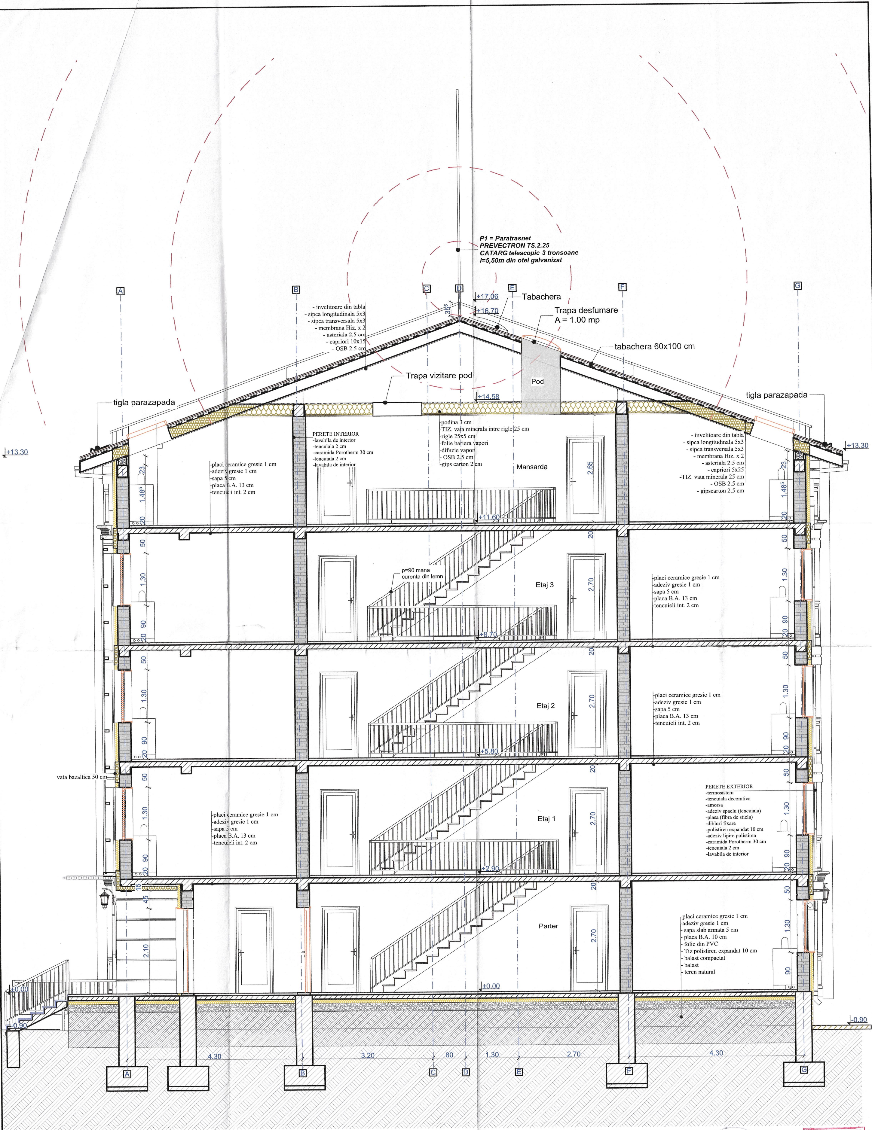
SECTIUNE A-A
