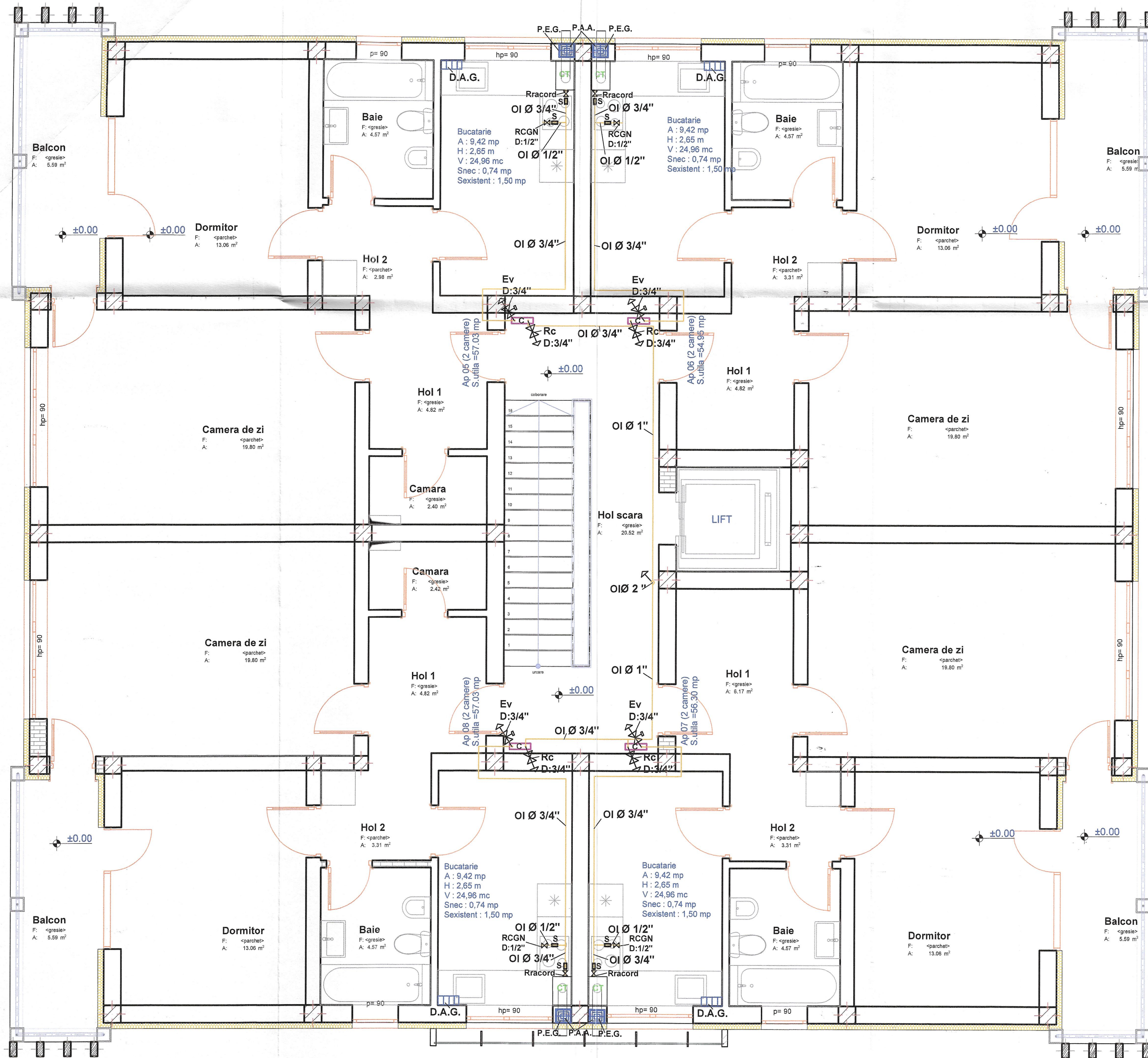
Plan etaj 1, etaj 2, etaj 3. Instalatii de utilizare gaze naturale. Scara 1:50
