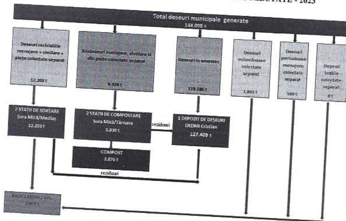
SCHEMA FLUXULUI DE DEȘEURI MUNICIPALE COLECTATE - 2023
