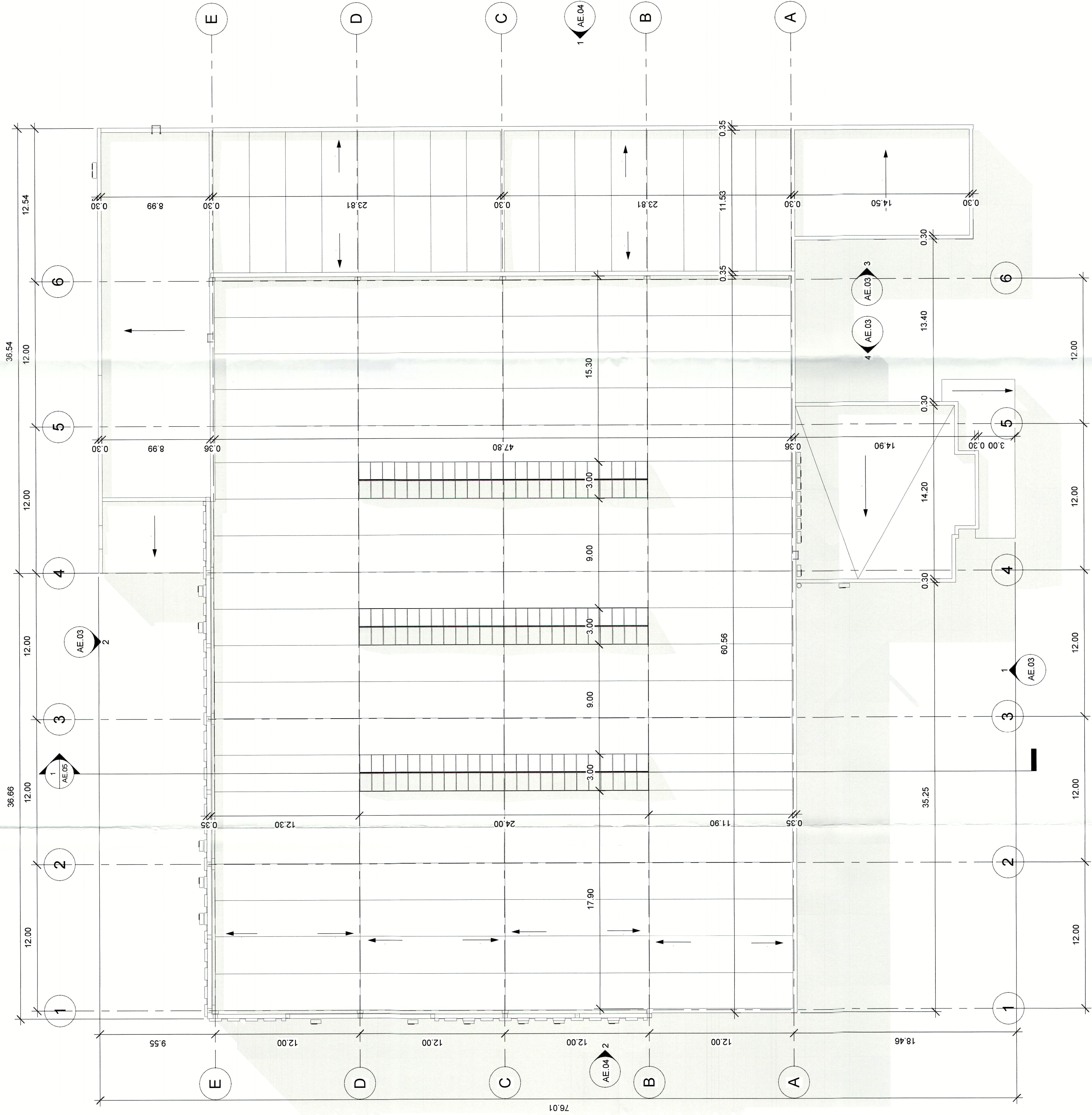
1 Plan Invelitoare 1 : 200
