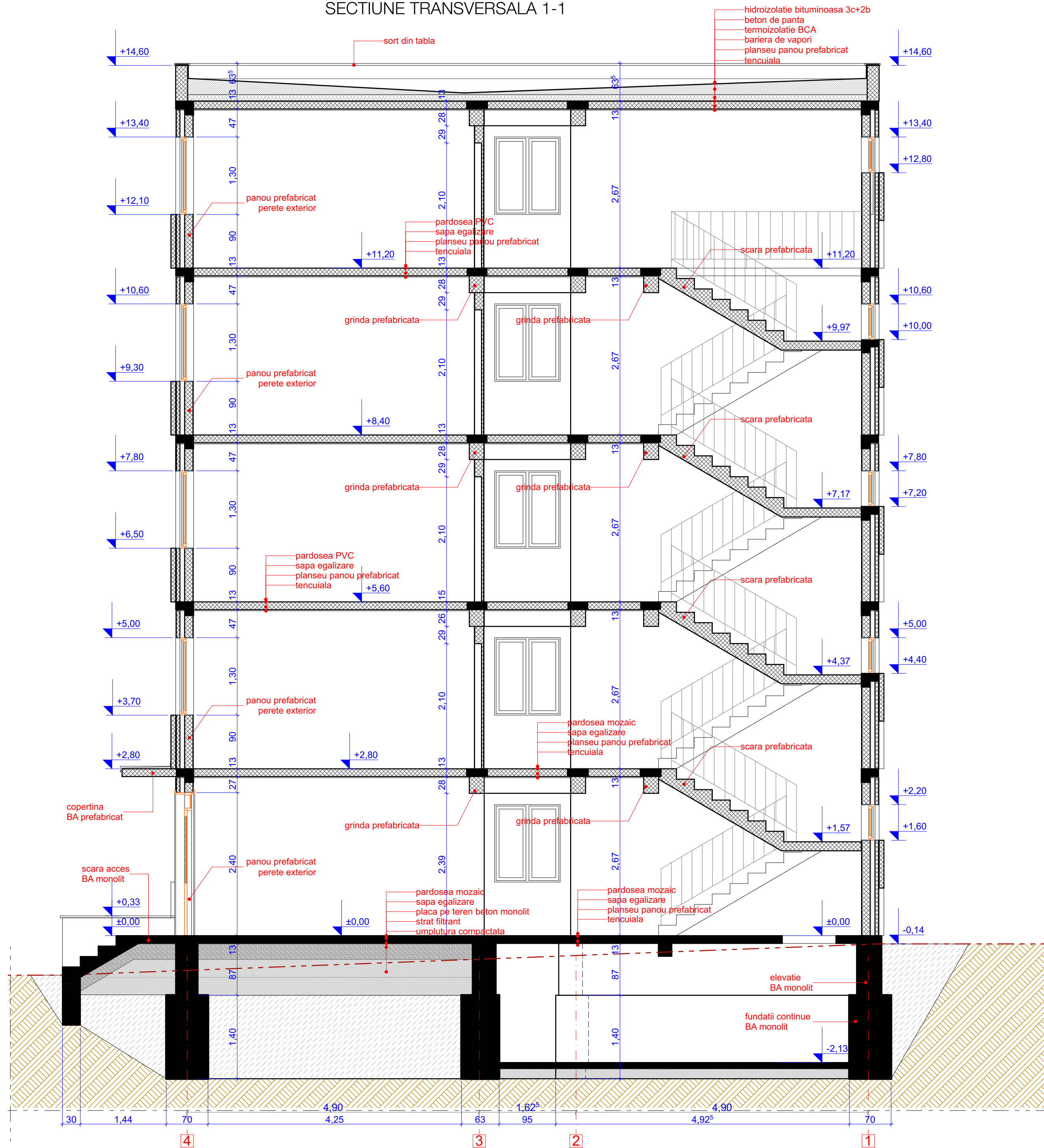
SECTIUNE TRANSVERSALA 1-1
