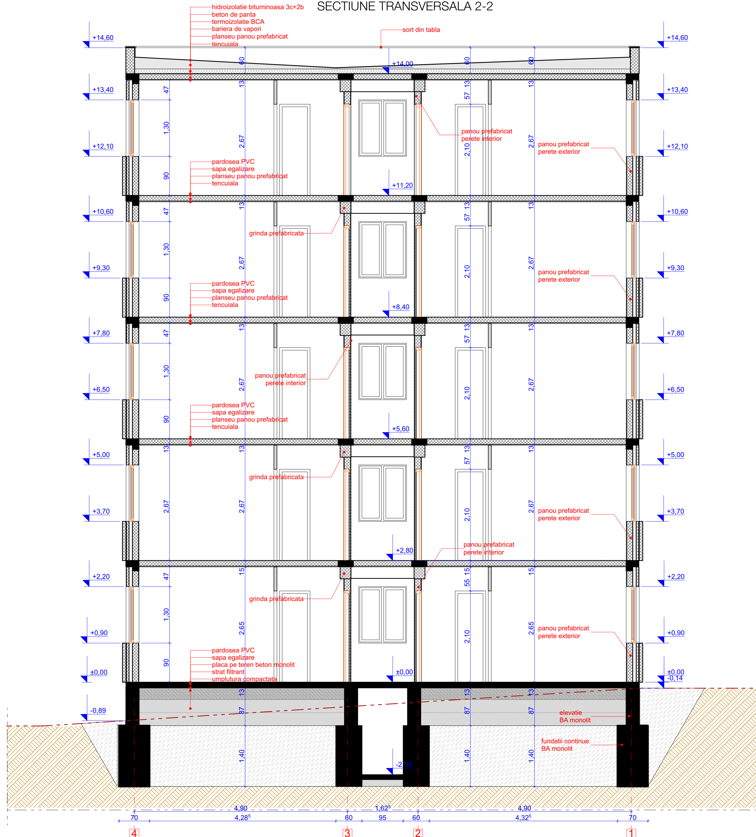
SECTIUNE TRANSVERSALA 2-2
