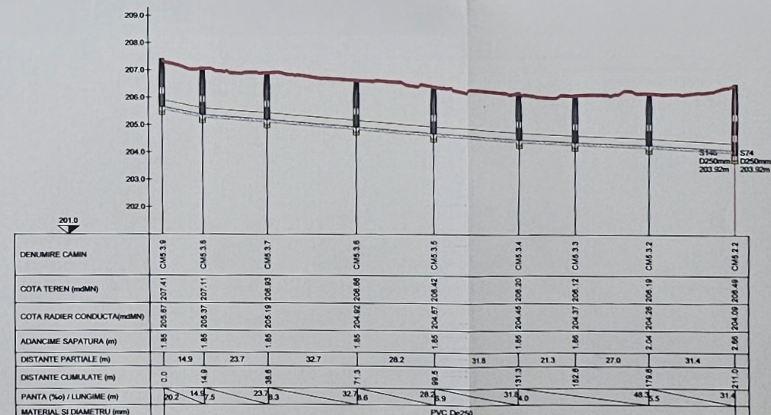
PROFIL LONGITUDINAL-Str. Lamaitei
