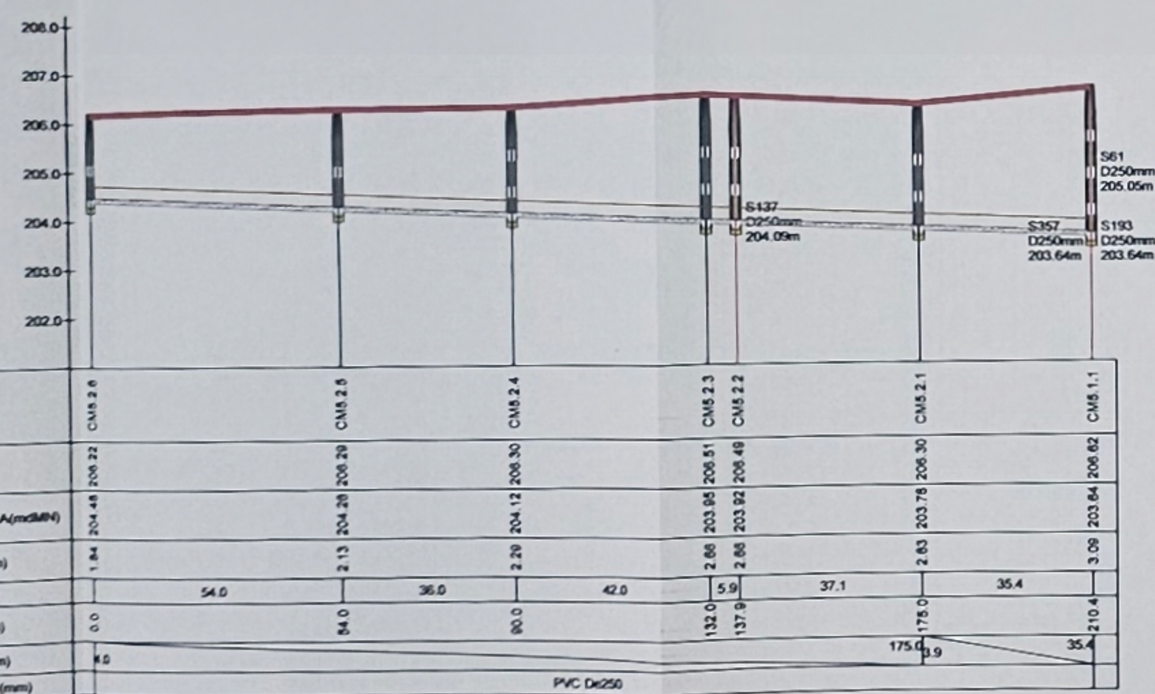
PROFIL LONGITUDINAL-Str. Garoafei 2
