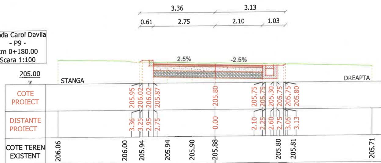
strada Carol Davila - P12 - km 0+240.00 Scara 1:100
