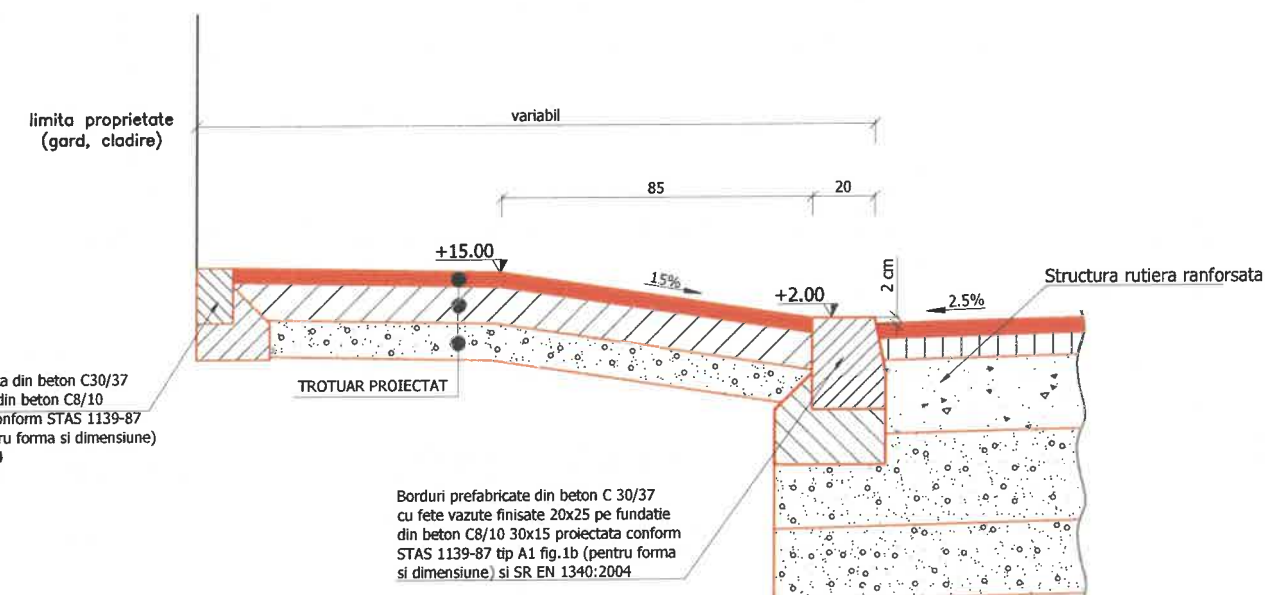
SECTIONE C-C Sc: 1:20
