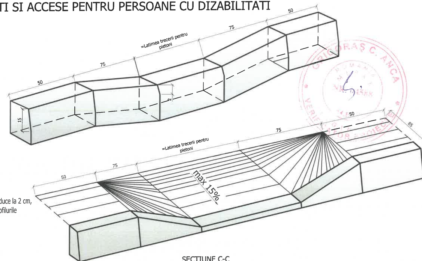
SECTIONE C-C Sc: 1:20
