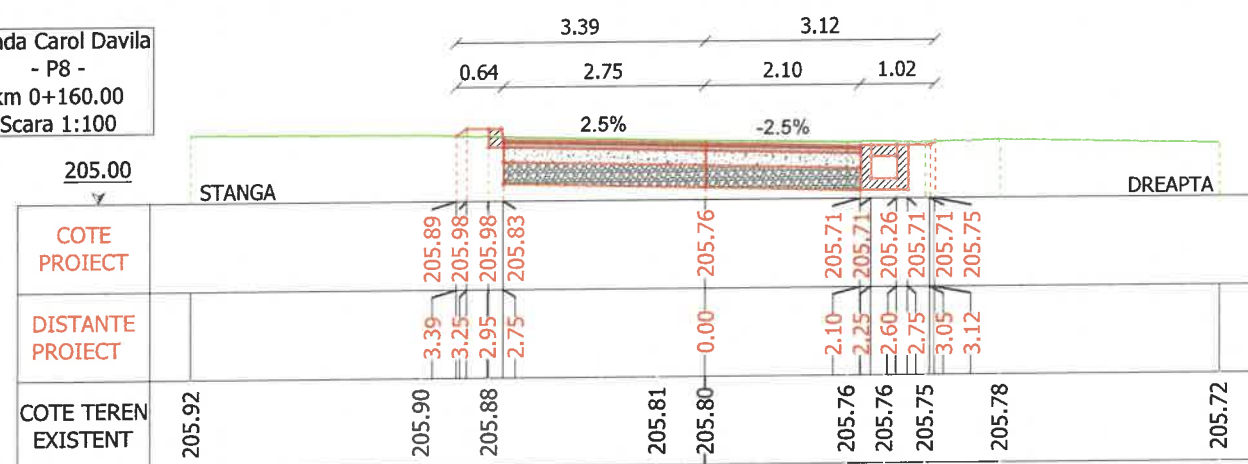
strada Carol Davila - P11 - km 0+220.00 Scara 1:100
