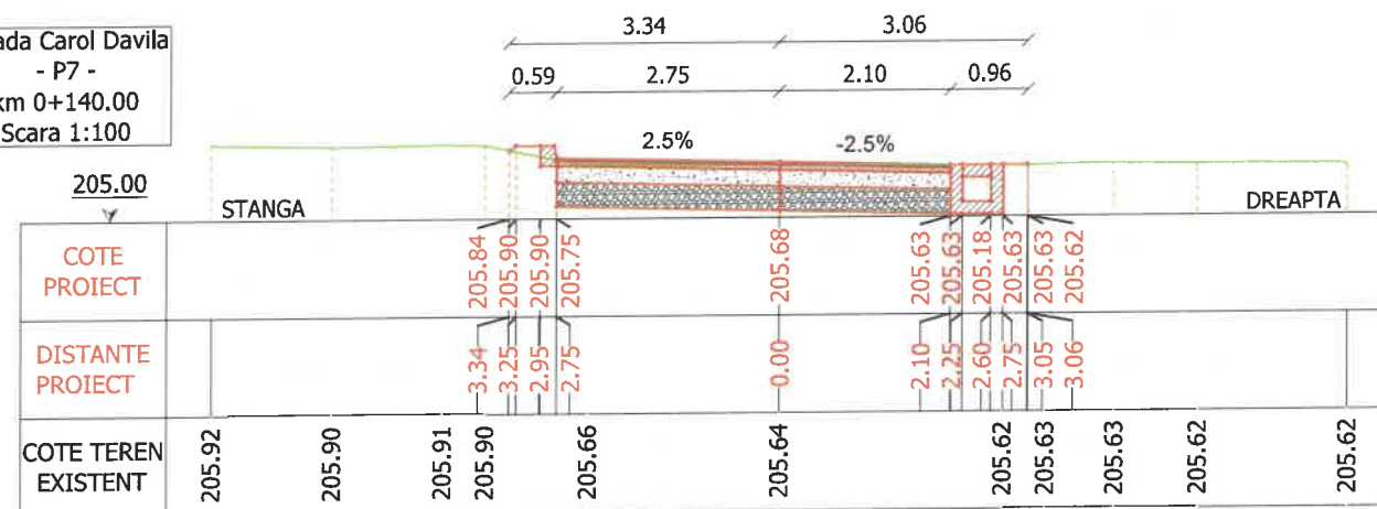
strada Carol Davila - P10 - km 0+200.00 Scara 1:100
