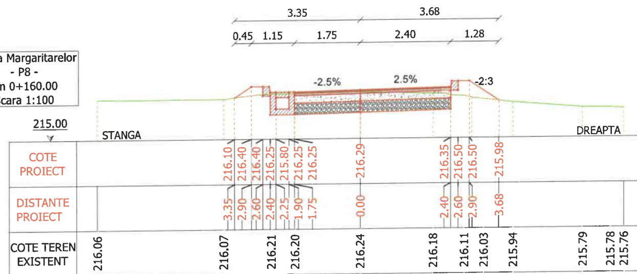
strada Margaritarelor - P11 - km 0+220.00 Scara 1:100
