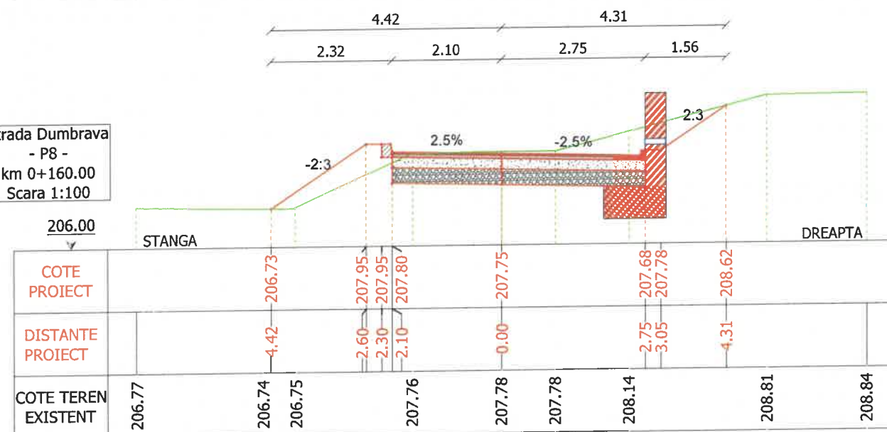
strada Dumbrava - P10 - km 0+200.00 Scara 1:100
