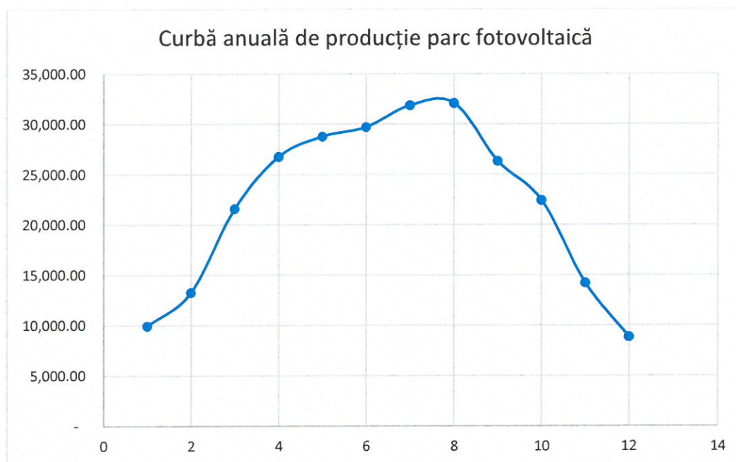
Fig. 2.2– Producție anuală, imobil 1 - CF 54082
