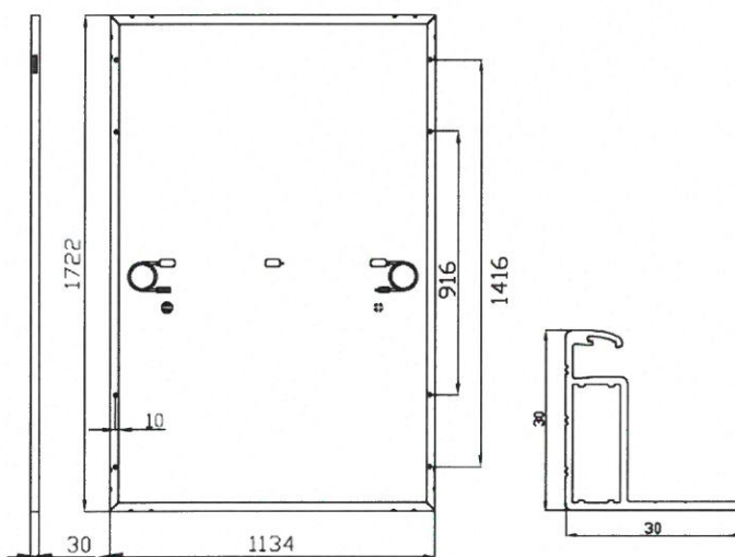
Fig.2.4 Panou fotovoltaic
