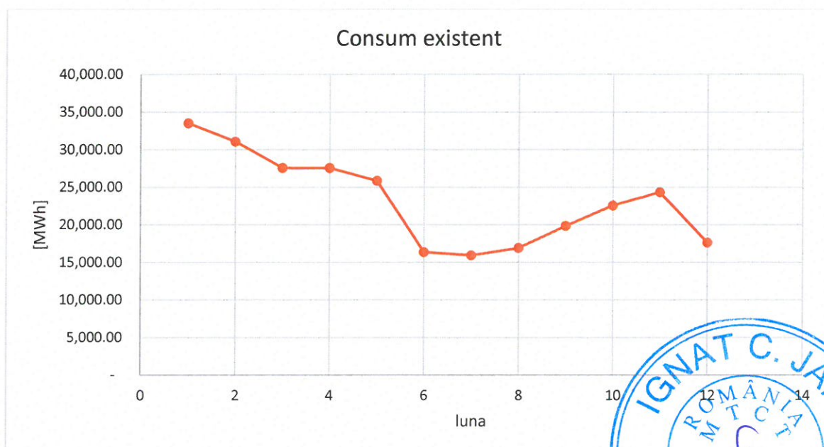
Fig. 2.1.–Consum anual - imobil 1- CF 54082
