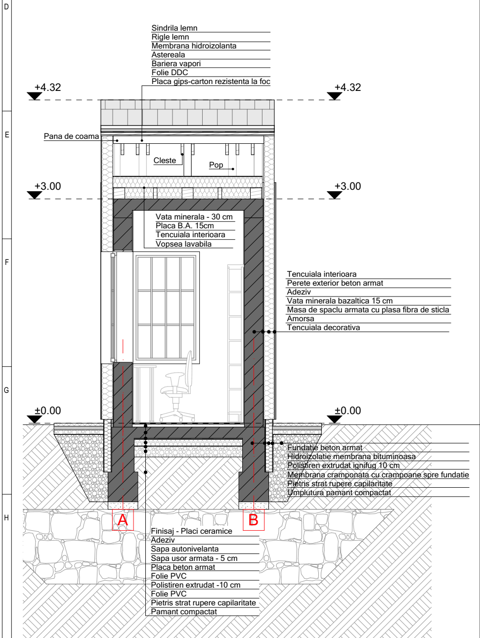
SECTIUNE LONGITUDINALA
