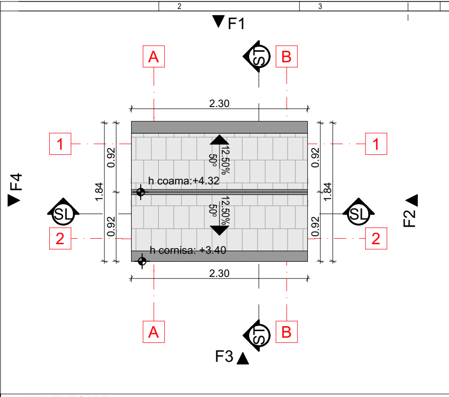
PLAN INVELITOARE
