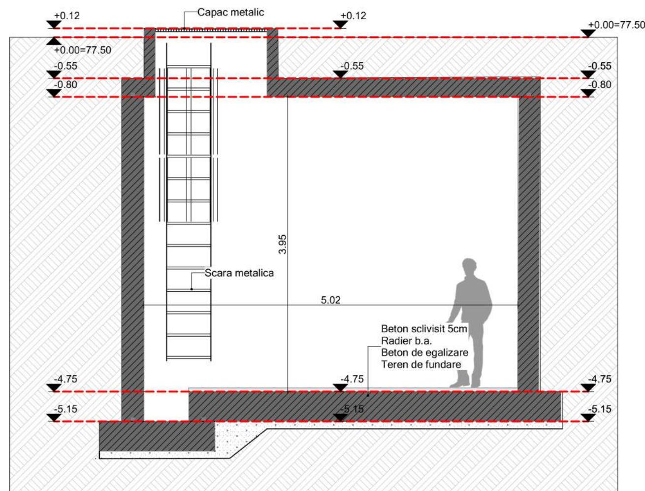
SECTIUNE SA
