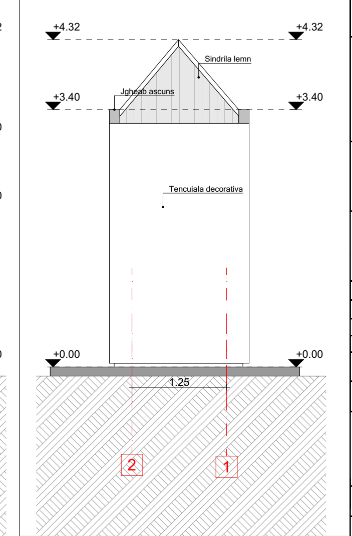
FATADA EST
