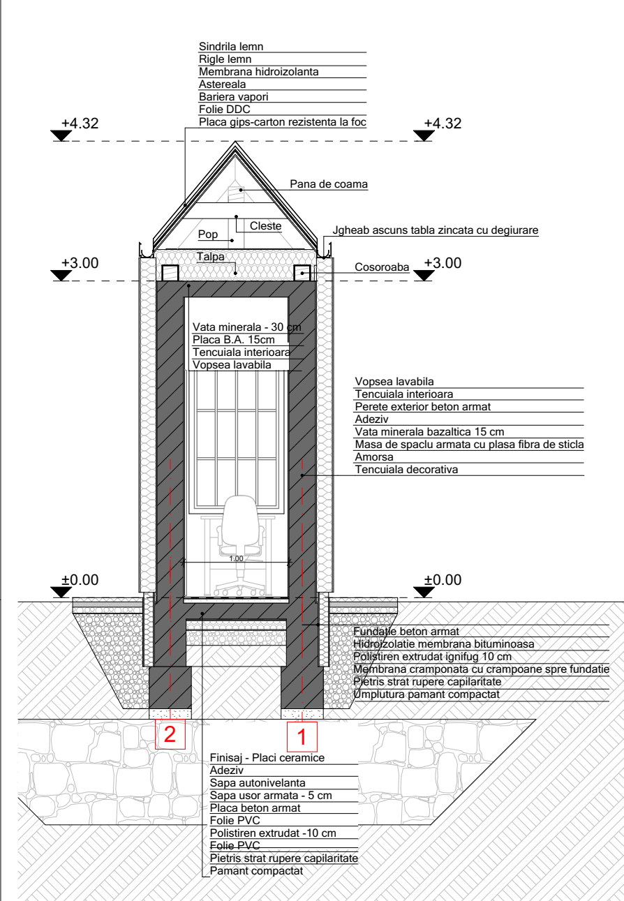
SECTIUNE TRANSVERSALA
