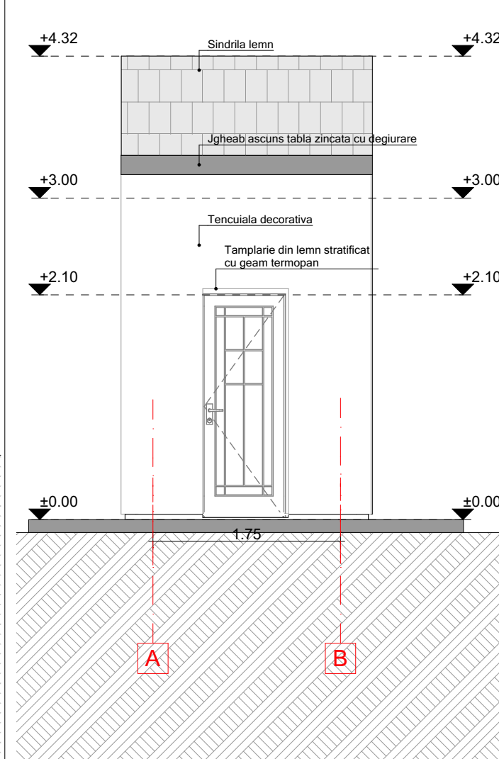
FATADA SUD
