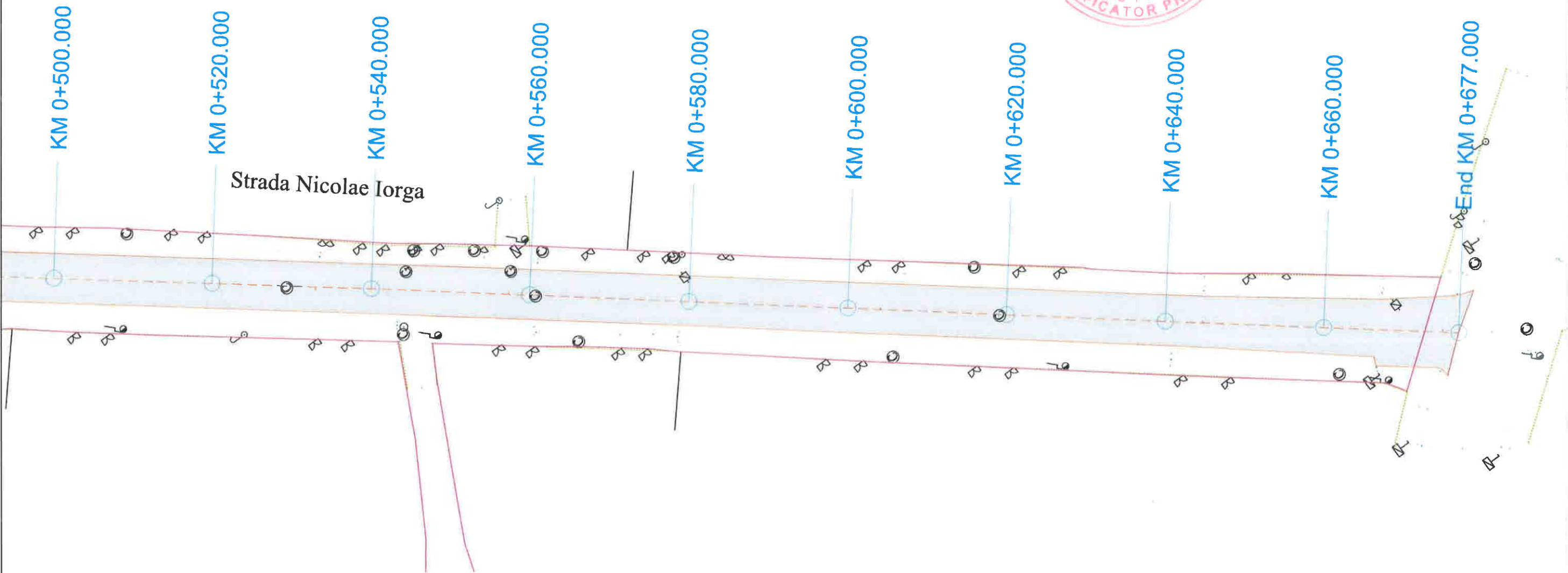
Detaliu SR Scara 1:20
