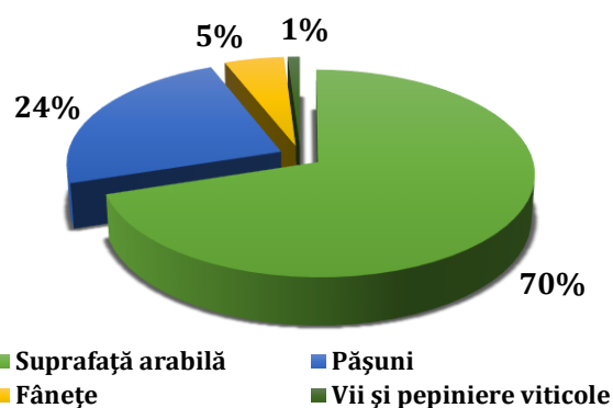
Fig. 3.2.3 Modul de utilizare al terenurilor agricole
