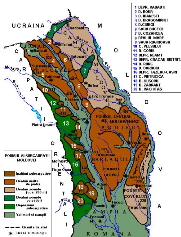
Fig. 2.2.1 Încadrarea geologică a comunei Tăcuta
