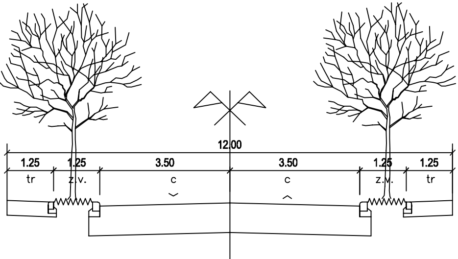
PROFIL TRANSVERSAL TIP - 12 M -
