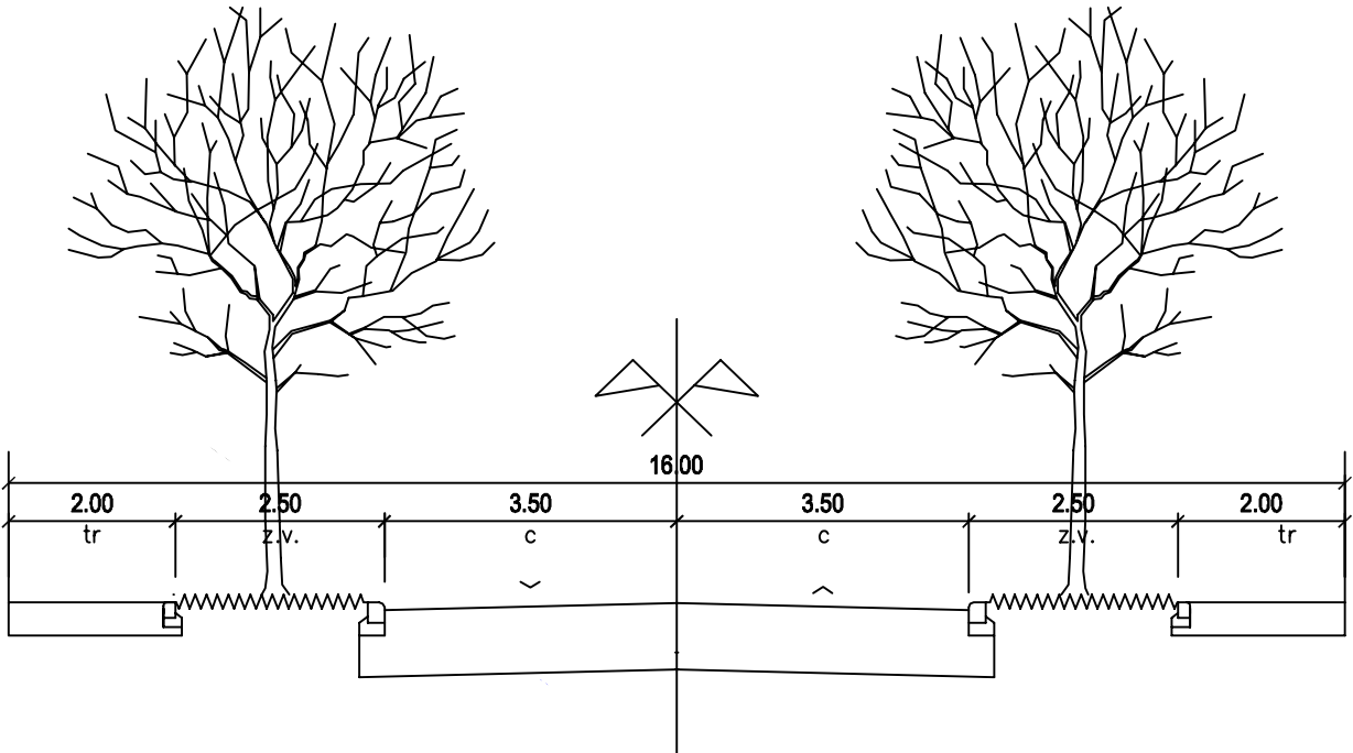
PROFIL TRANSVERSAL TIP - 16 M -
