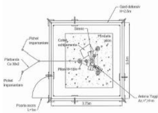
Fig. 6 - Pilon zăbreliț H=10-30m-vedere de sus
