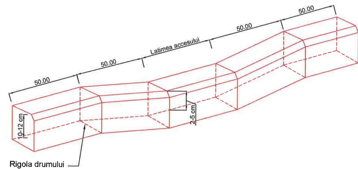
Detaliu C DETALIU AMENAJARE ACCES PROPRIETATI
