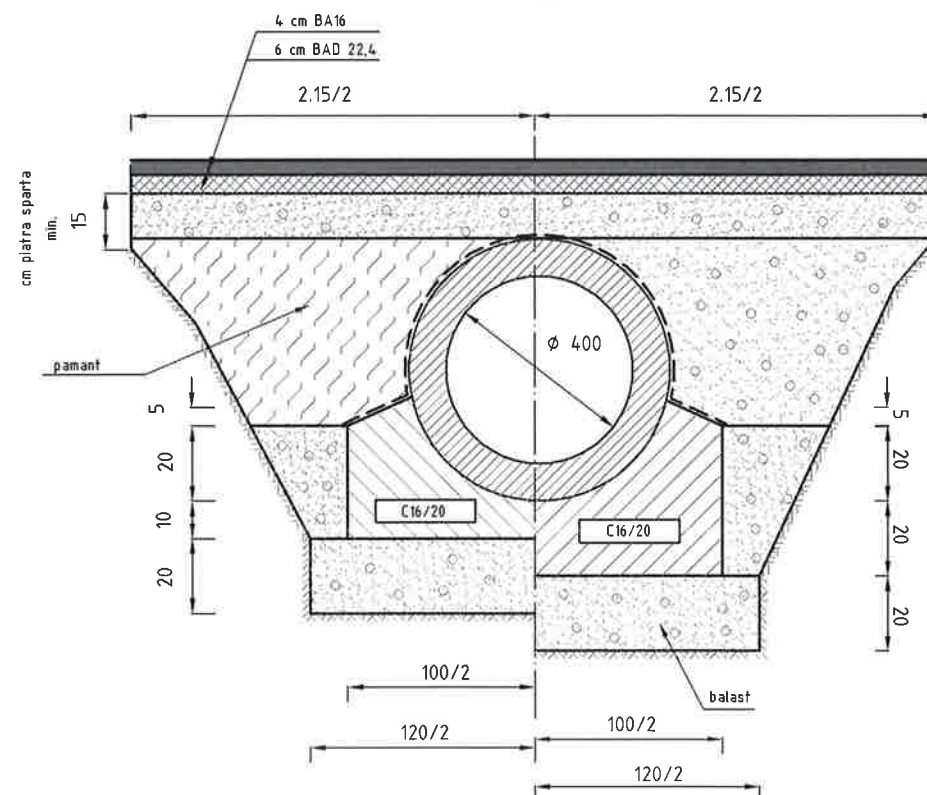
SECTIUNE C - C Sc 1:20
