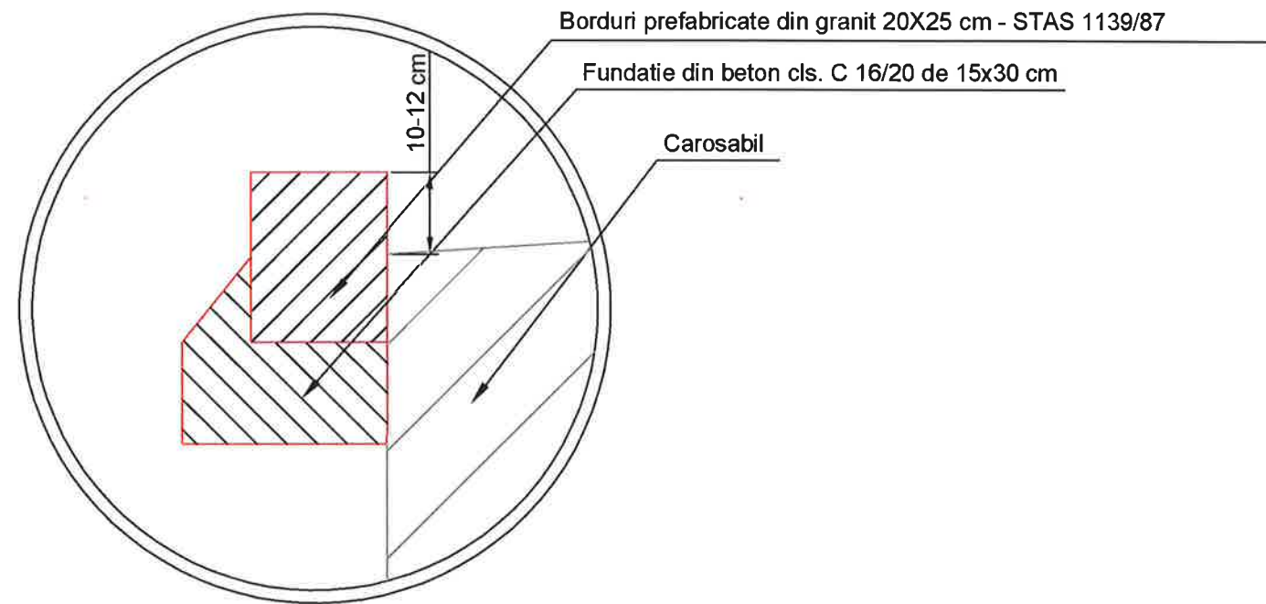
Detaliu A INCADRARE CAROSABIL
