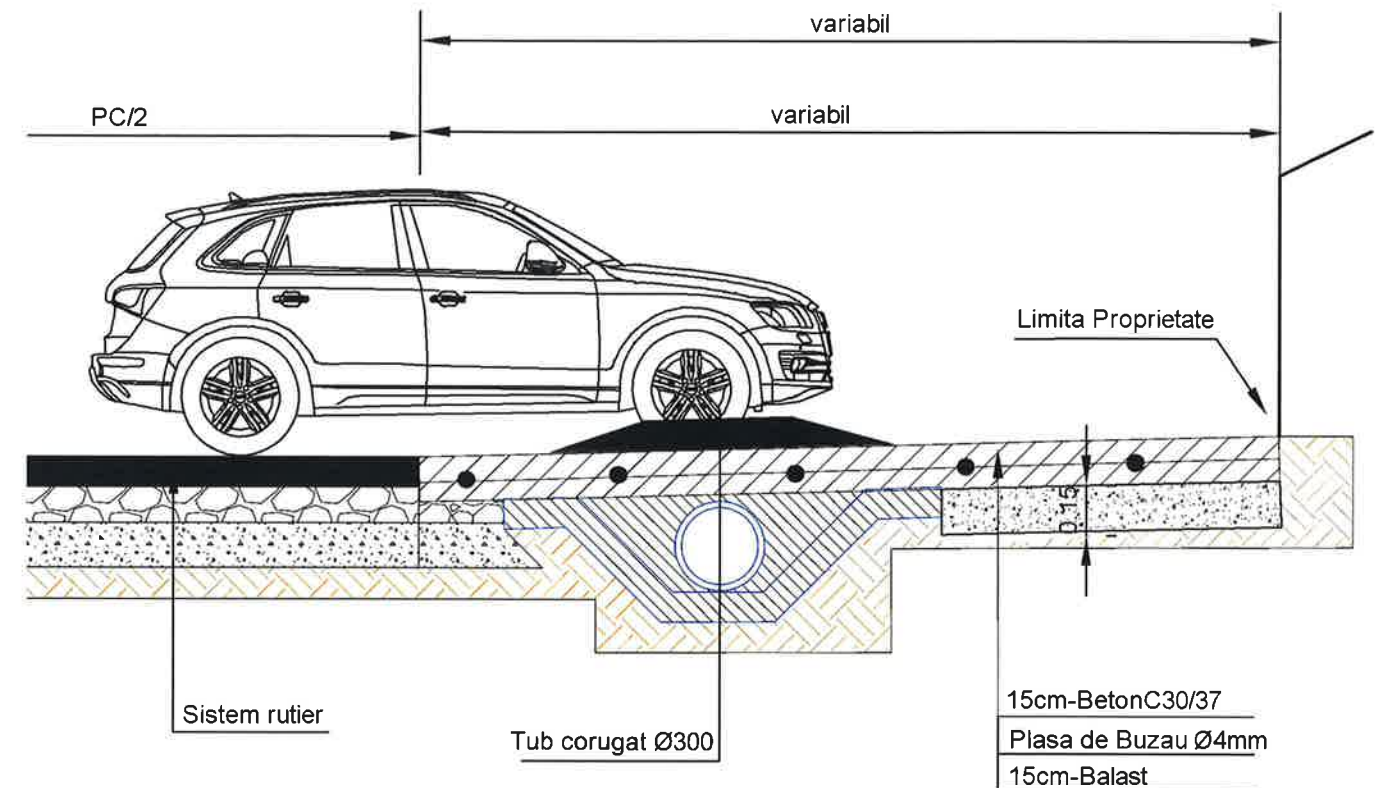
SECTIUNE A-A Scara 1:20
