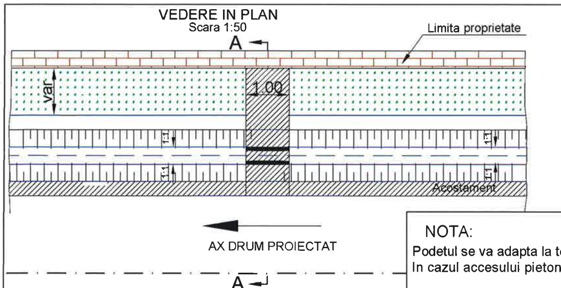
DETALIU ACCES PIETONAL LA PROPRIETATI - PESTE SANT
