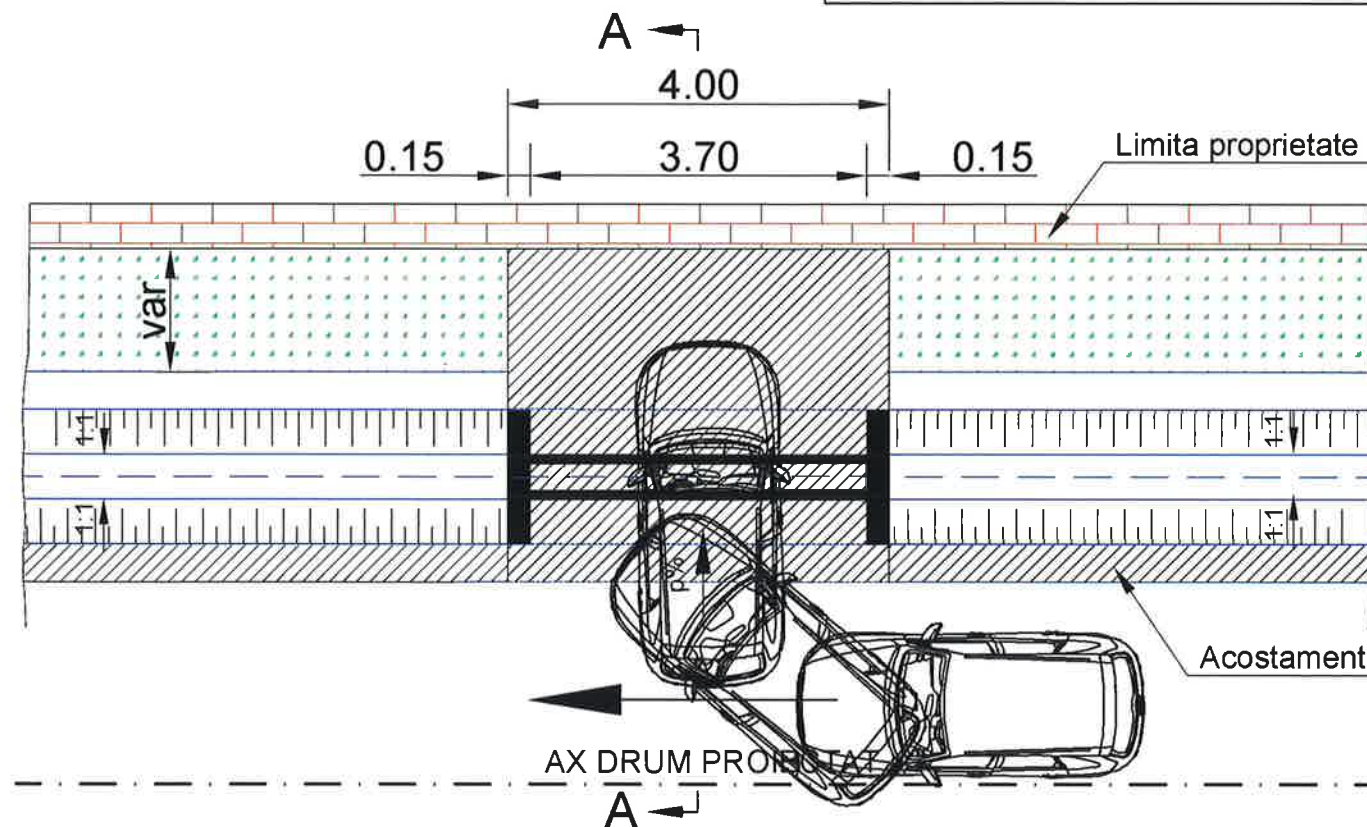
VEDERE IN PLAN Scara 1:50
