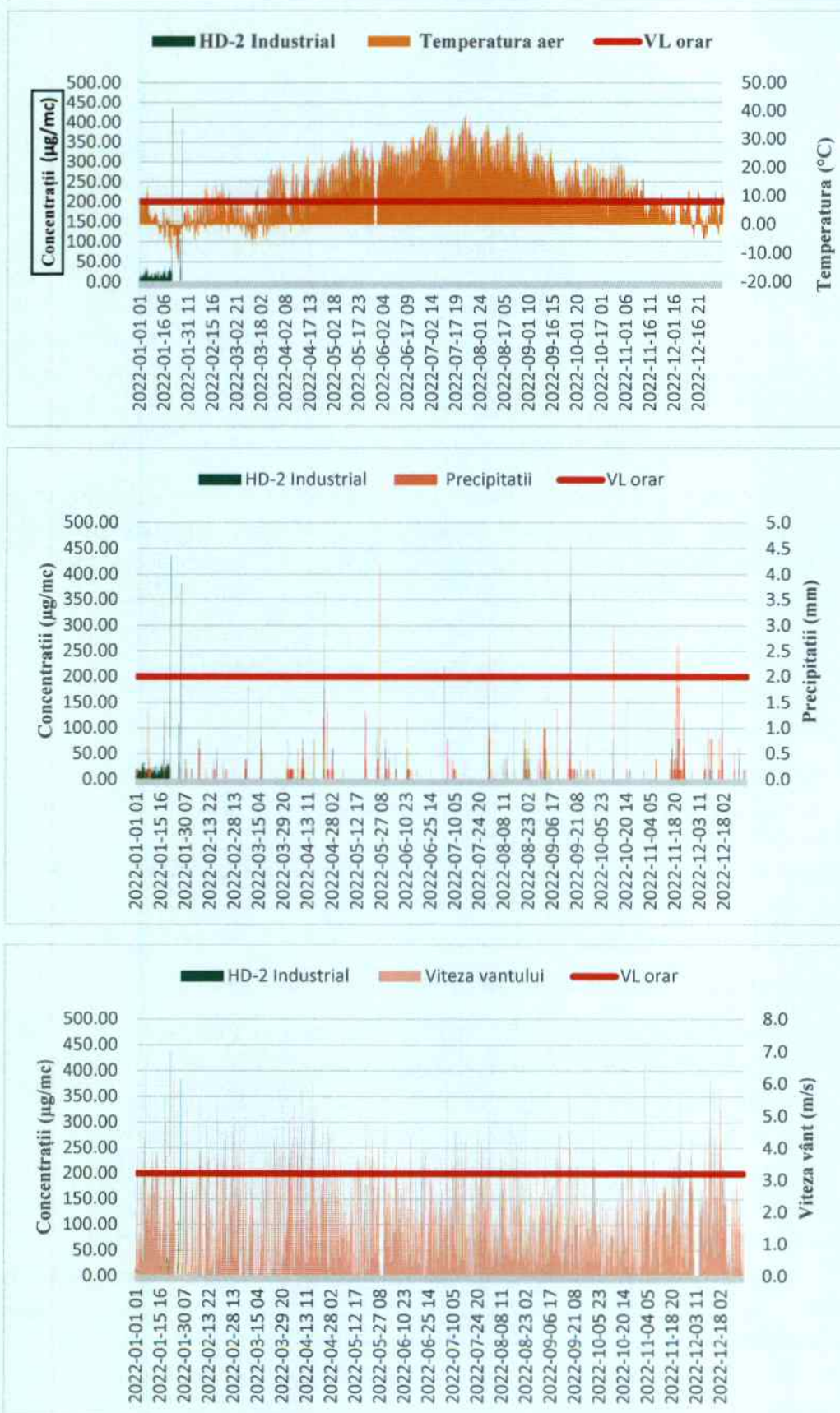
Figura nr. 3-14 Concentrații medii orare pentru dioxid de azot (NO 2 ) comparativ cu temperatura aerului, precipitațiile atmosferice și viteza vântului, înregistrate la stația HD-2, în anul 2022
