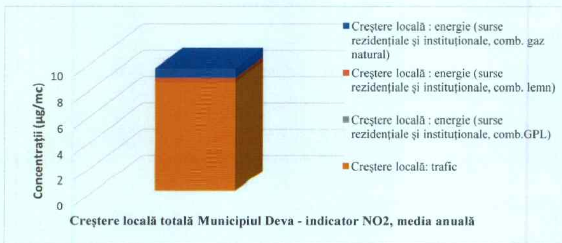
Figura nr. 5-9 Creșterea locală totală
