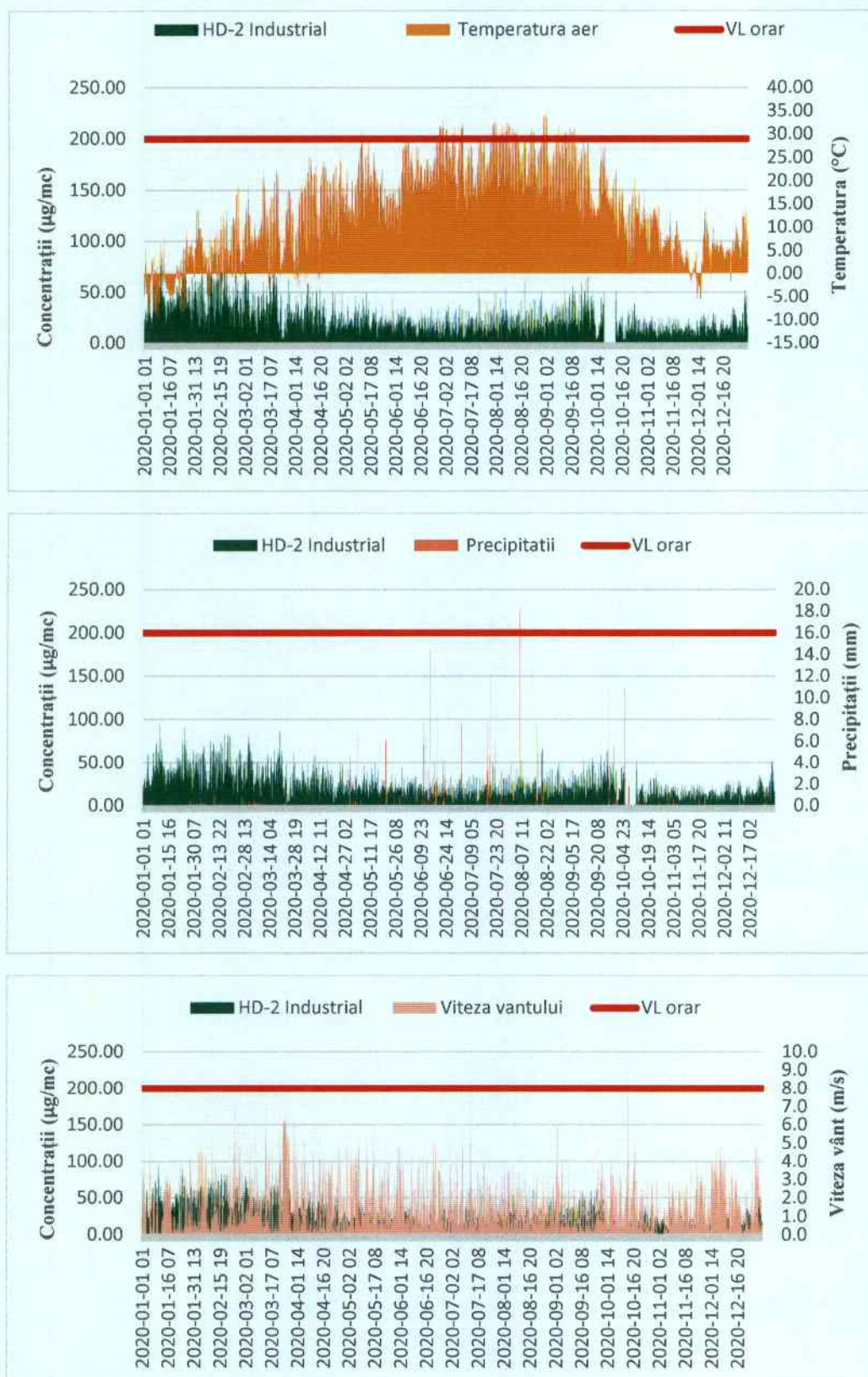
Figura nr. 3-12 Concentrații medii orare pentru dioxid de azot (NO 2 ) comparativ cu temperatura aerului, precipitațiile atmosferice și viteza vântului, înregistrate la stația HD-2, în anul 2020
