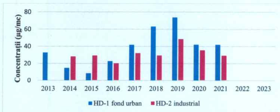
Figura nr. 3-2 Tendința concentrației medii anuale pentru oxizii de azot (NO x ) (µg/mc), înregistrată la stațiile automate de monitorizare din municipiul Deva, în perioada 2013 -2023
