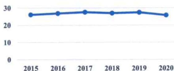
Număr mediu anual de zile senine
