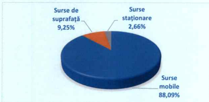
Figura nr. 4-2 Pondere emisiilor de NO x , pe categorii de surse, în municipiul Deva
