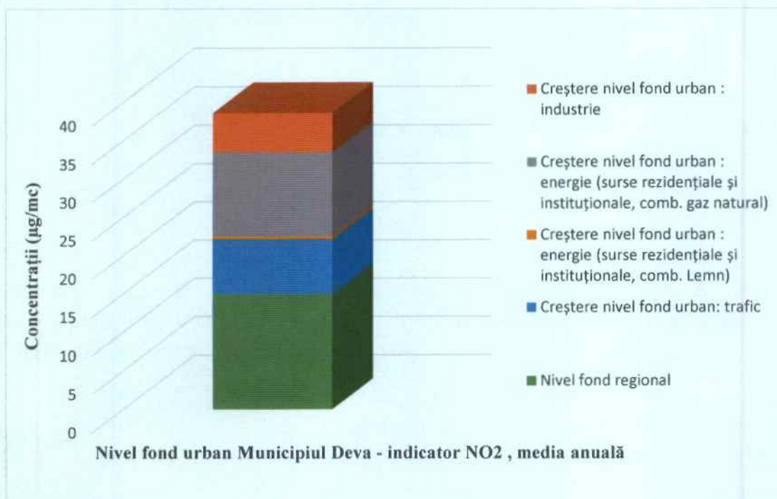
Figura nr. 5-10 Nivel fond urban total – indicator NO 2
