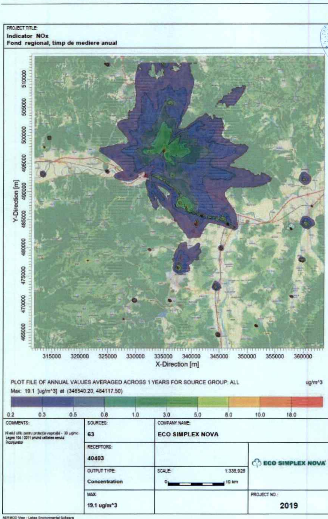
Figura nr. 5-2 Fond regional total municipiul Deva, indicator NO x , perioada de mediere anual, an referință 2019
