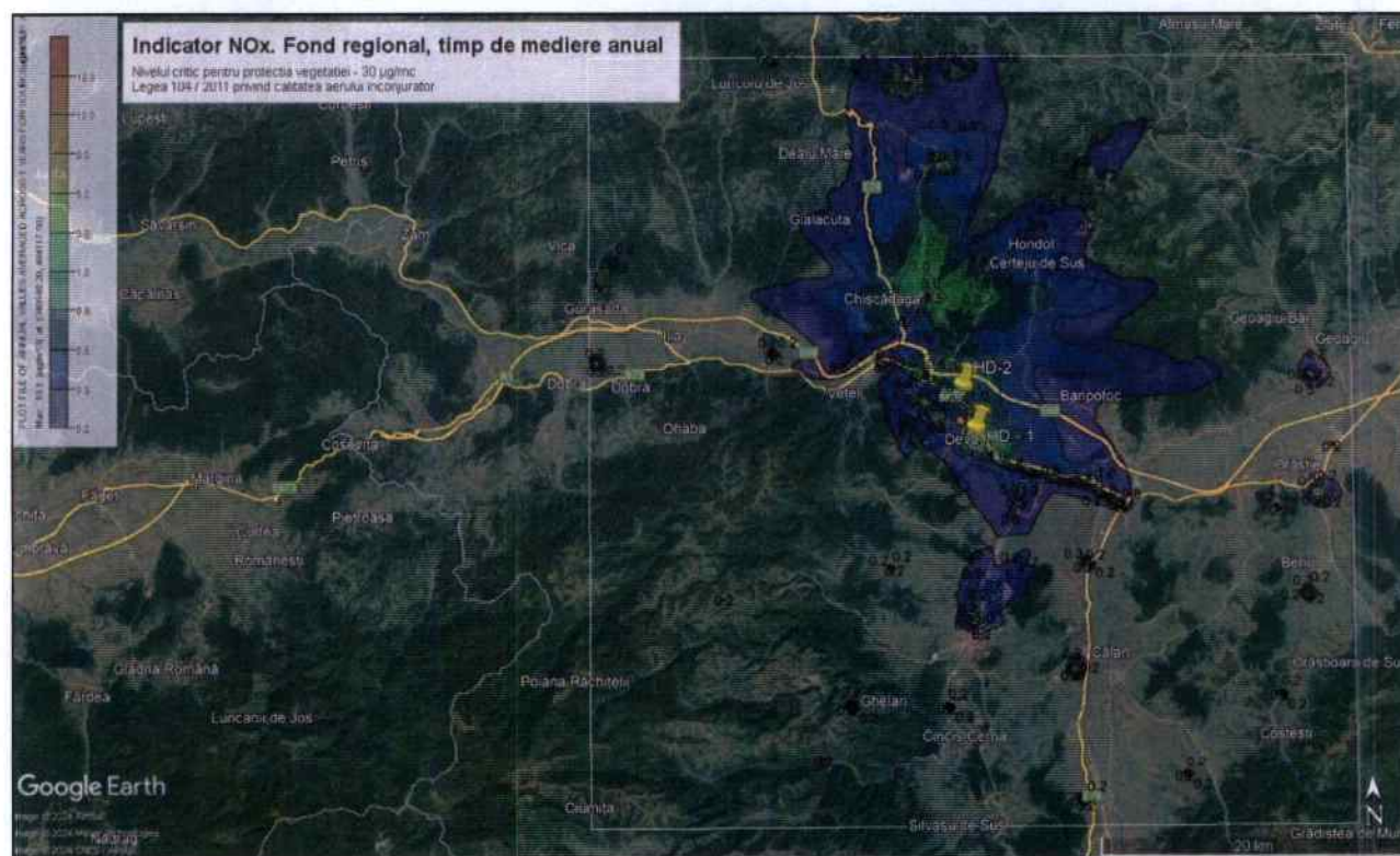
Figura nr. 5-3 Fond regional indicator NO 2 / NO x , perioada de mediere anual, an referință 2019
