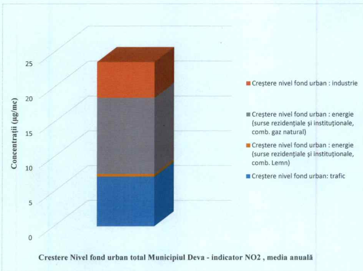
Figura nr. 5-4 Creștere nivel fond urban total municipiul Deva – indicator NO 2 , media anuală
