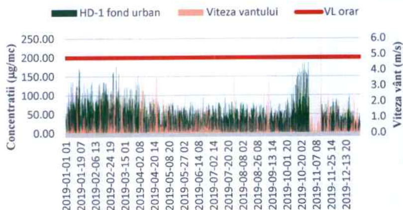
Figura nr. 3-7 Concentrații medii orare pentru dioxid de azot (NO 2 ) comparativ cu temperatura aerului, precipitațiile atmosferice și viteza vântului, înregistrate la stația HD-1, în anul 2019
