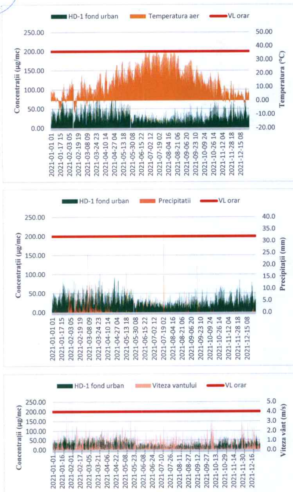
Figura nr. 3-9 Concentrații medii orare pentru dioxid de azot (NO 2 ) comparativ cu temperatura aerului, precipitațiile atmosferice și viteza vântului, înregistrate la stația HD-1, în anul 2021
