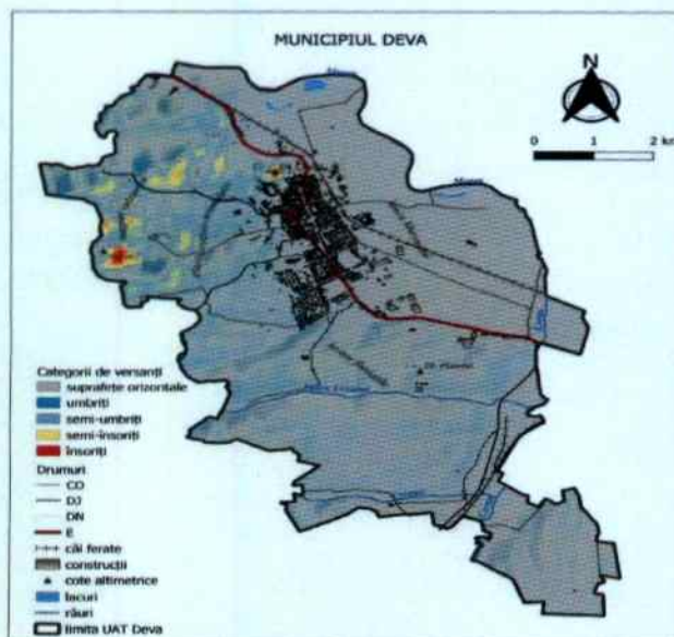
Figura nr. 2-35 Harta orientării versanților
