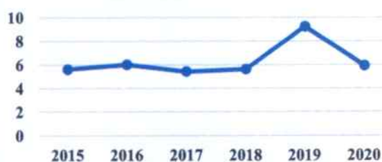
Nebulozitatea medie anuală (zecimi)
