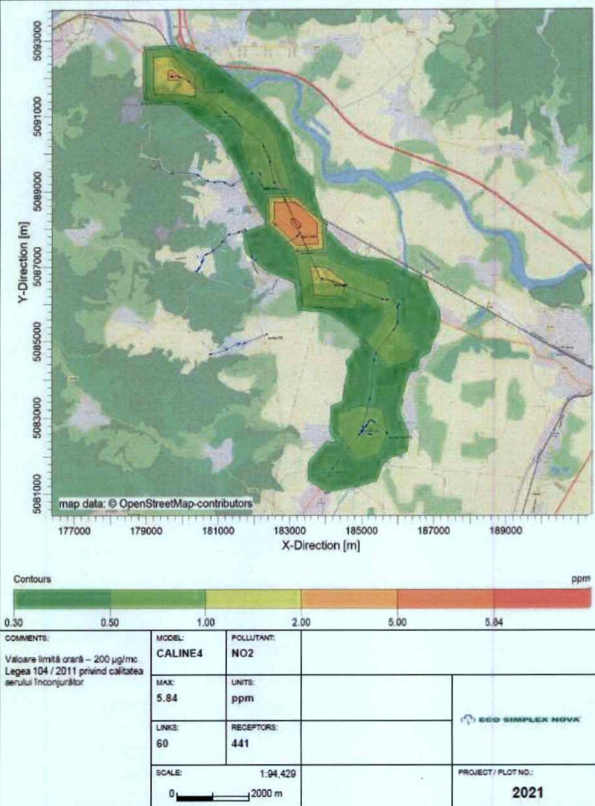
Figura nr. 5-8 Creșterea nivelului de fond urban – MUNICIPIUL DEVA – trafic rutier – oră de vârf - indicator NO 2 , perioada de mediere 1 oră, an referință 2019
