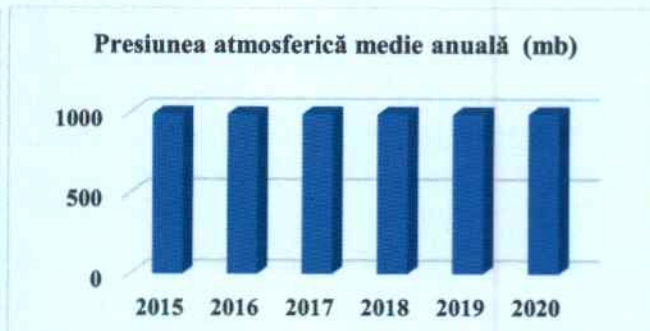
Figura nr. 2-21 Presiunea atmosferică medie anuală
