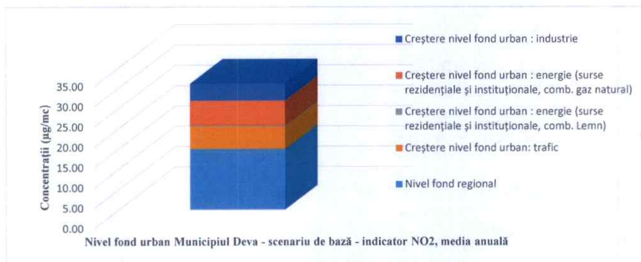
Figura nr. 6-1 Nivel fond urban total Municipiul Deva, an proiecție – scenariu de bază – indicator NO 2 , media anuală
