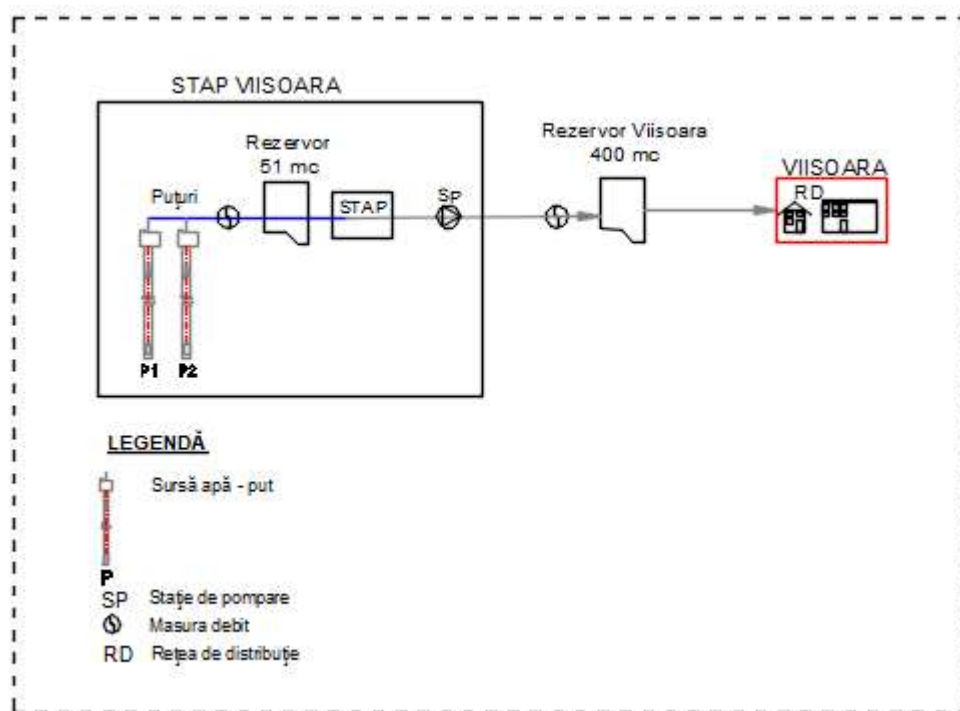
Figura Error! No text of specified style in document. -67 - Schema sistemului de alimentare cu apa SAA Viisoara
