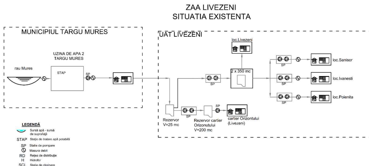
Figura Error! No text of specified style in document.-24 – Schema sistem apa potabila din ZAA Targu Mures – Livezeni
