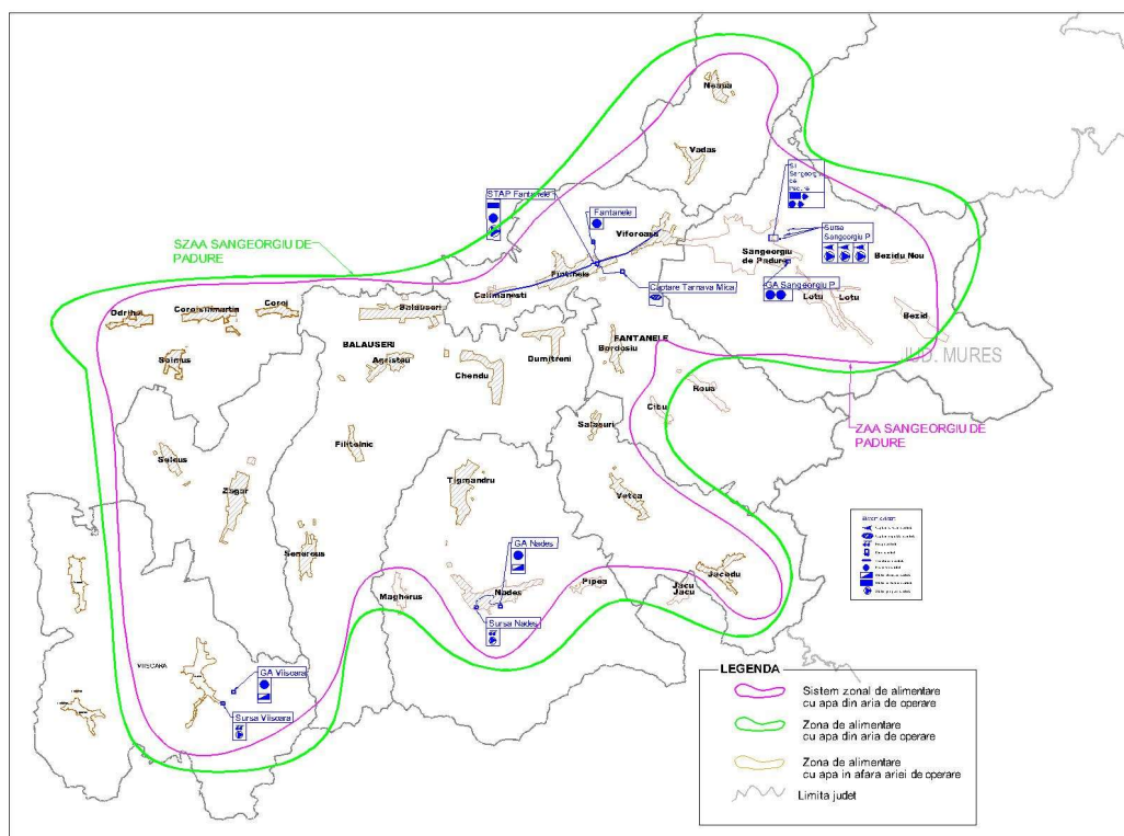
Figura Error! No text of specified style in document.-61 - Incadrarea in zona a sistemului zonal de alimentare cu apa SZAA Sangeorgiu de Padure
