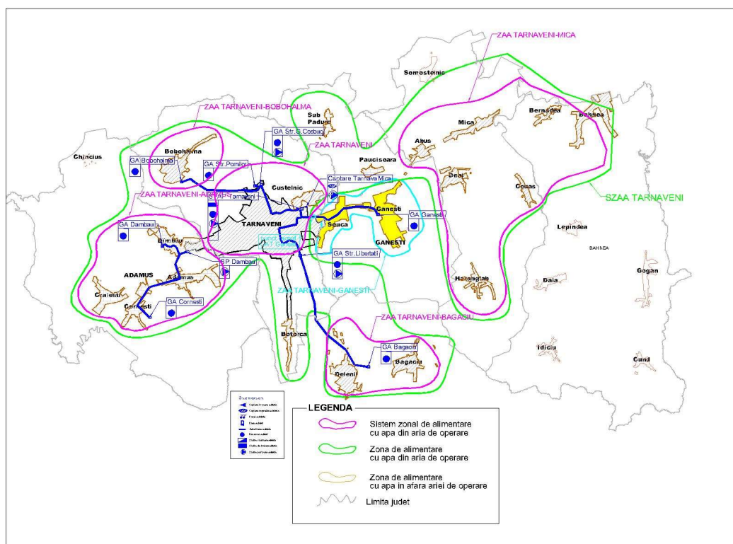
Figura Error! No text of specified style in document.-55 Incadrarea în zona a sistemului zonal de alimentare cu apă SZAA Tarnaveni
