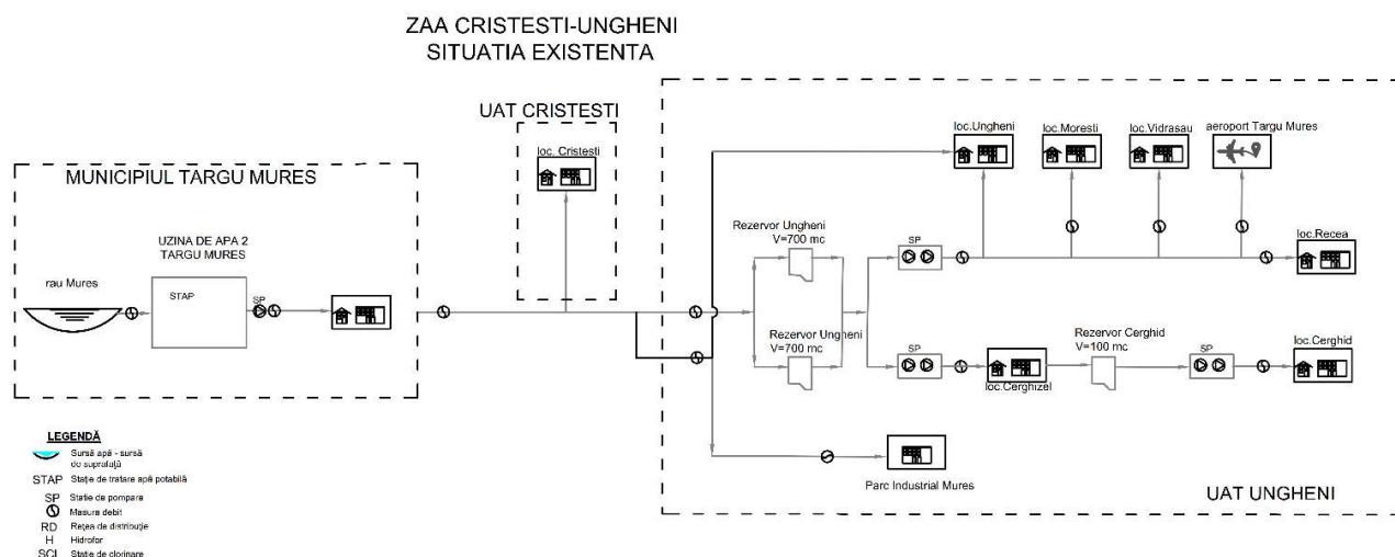
Figura Error! No text of specified style in document. -28 – Schema conductelor de transport apa potabila din ZAA Targu Mures – Cristești-Ungheni
