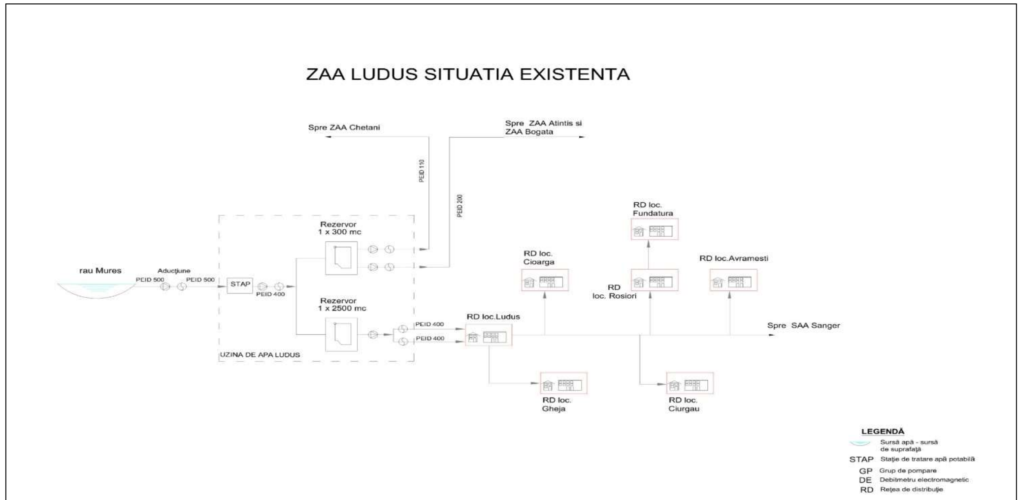
Figura Error! No text of specified style in document. -48 - Schema zonei de alimentare cu apa Ludus existenta 2021
