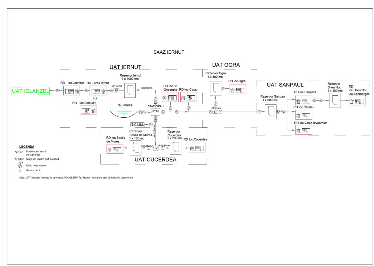
Figura Error! No text of specified style in document.-79 - Schema sistemului zonal de alimentare cu apa SZA Iernut
