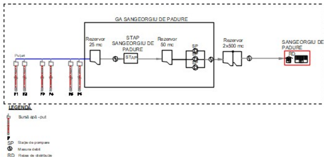
Figura Error! No text of specified style in document.-62 - Schema sistemului de alimentare cu apa Sangeorgiu de Padure
