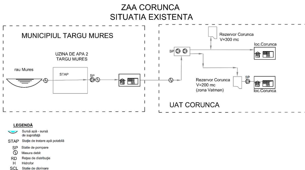
Figura Error! No text of specified style in document. -26 – Schema sistem apă potabilă din ZAA Corunca
