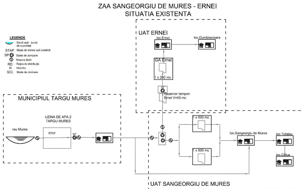
Figura Error! No text of specified style in document. -22 - Schema zona de alimentare cu apa potabila ZAA Targu Mures – Sângeorgiu de Mures - Ernei
