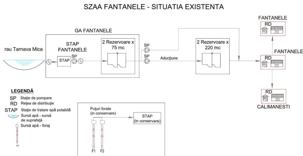
Figura Error! No text of specified style in document. -64 - Schema sistemului de alimentare cu apa SAA Fantanele
