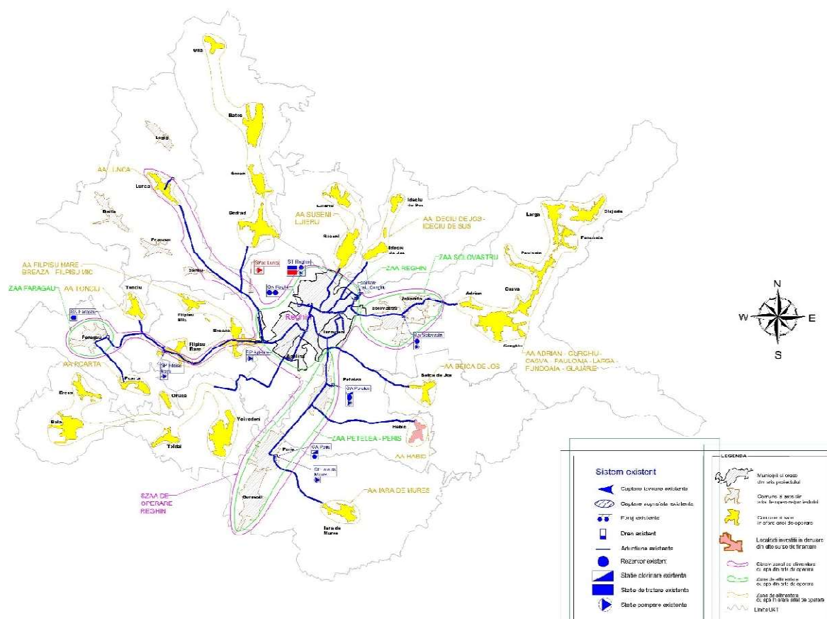
Figura Error! No text of specified style in document. -34 - Incadrarea in zona a sistemului zonal de alimentare cu apa Reghin
