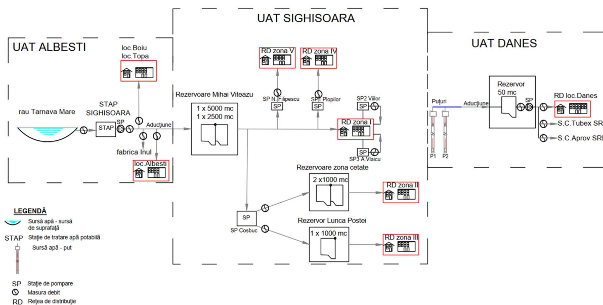
Figura Error! No text of specified style in document.-70 - Schema sistemului zonal de alimentare cu apa SZAA Sighisoara
