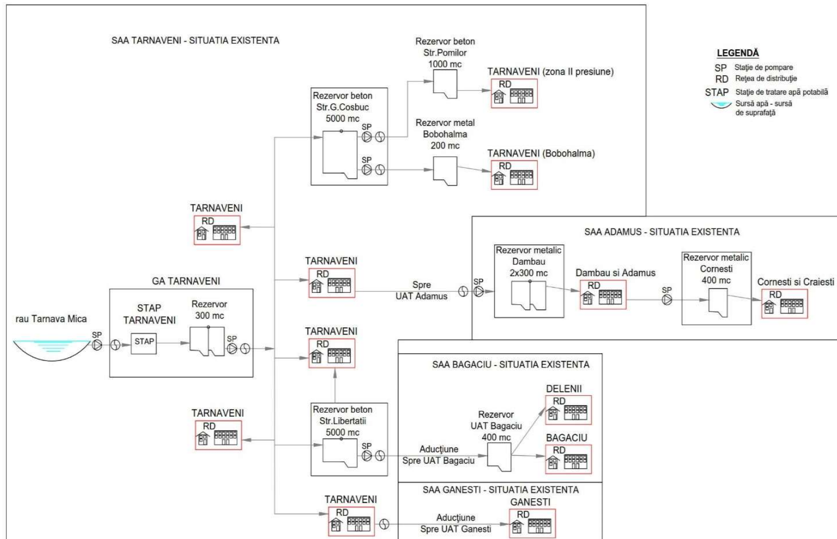
Figura Error! No text of specified style in document.-56 - Schema sistemului de alimentare cu apă SZAA Tarnaveni
