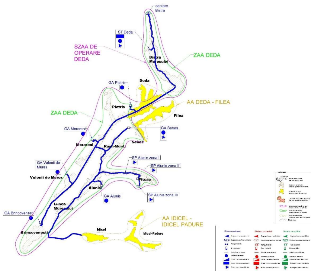
Figura Error! No text of specified style in document.-81 - Incadrarea in zona a sistemului zonal de alimentare cu apa Deda
