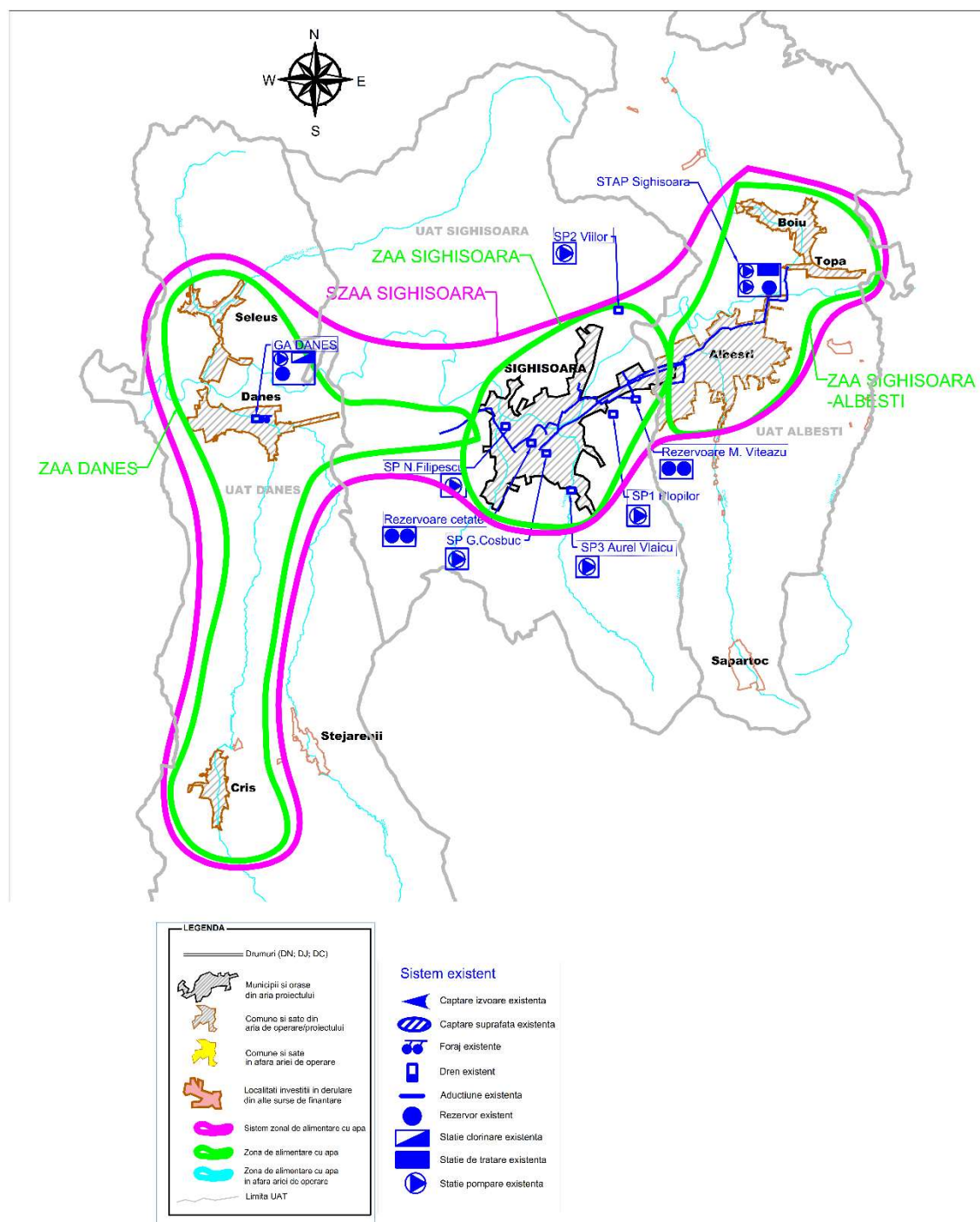
Figura Error! No text of specified style in document.-69 - Incadrarea în zona a sistemului zonal de alimentare cu apă SZAA Sighisoara
