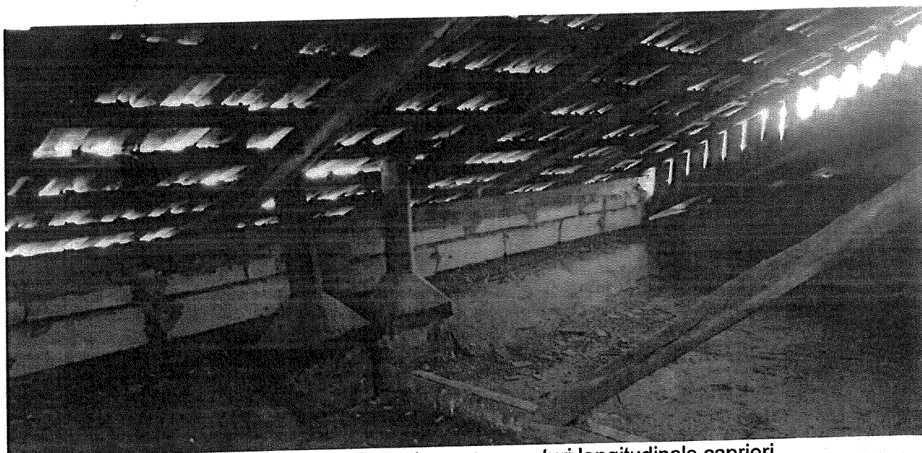
Pop si pana longitudinală – crapaturi longitudinale + noduri nesolidarizate
