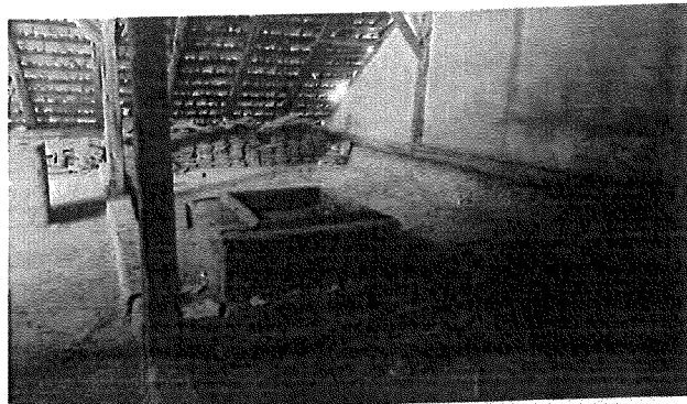
Ziduri frontoane - lipsa centuri si stalpisori de confinare
