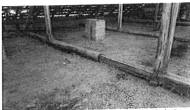
Lipsa ancorare talpi in elementele de beton ale structurii + asezare elemente de rezistenta ale sarpantei direct pe termo-hidroizolatia existenta (zgura + termoizolatatie zgura + hidroizolatatie)
