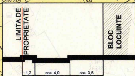
ALEE - din strada Arad PROFIL EXISTENT SI MENTINUT
