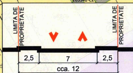
STRADA ARAD PROFIL EXISTENT / MENTINUT
