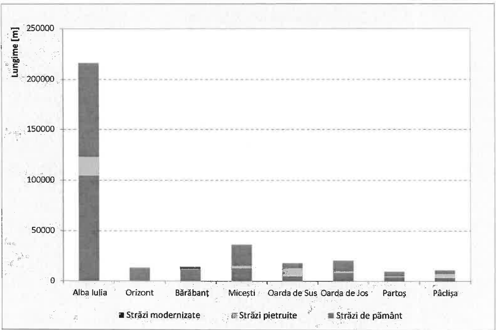
Fig.3 Lungimea străzilor în funcție de tipul îmbrăcămînții (sursa: PMUD al mun. Alba Iulia) Proporția de 44% a străzilor modernizate înseamnă imbrăcăminte din: asfalt, asfalt/beton, pavaj bazalt sau pavaj beton.
