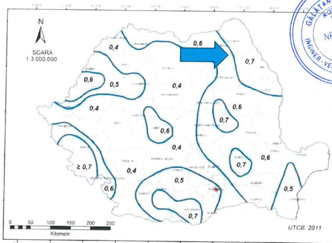
Fig.3.5 – Zonarea Teritoriului din punct de vedere al presiunii vântului
