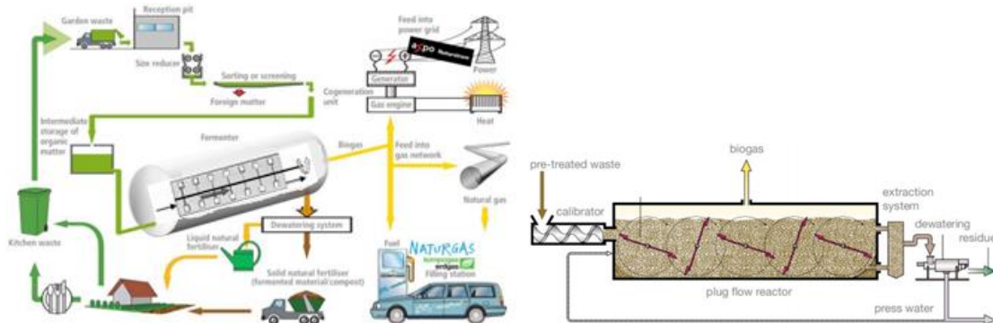
Figură 3-7 – Digestie anaerobă semi-uscă (exemplu)
