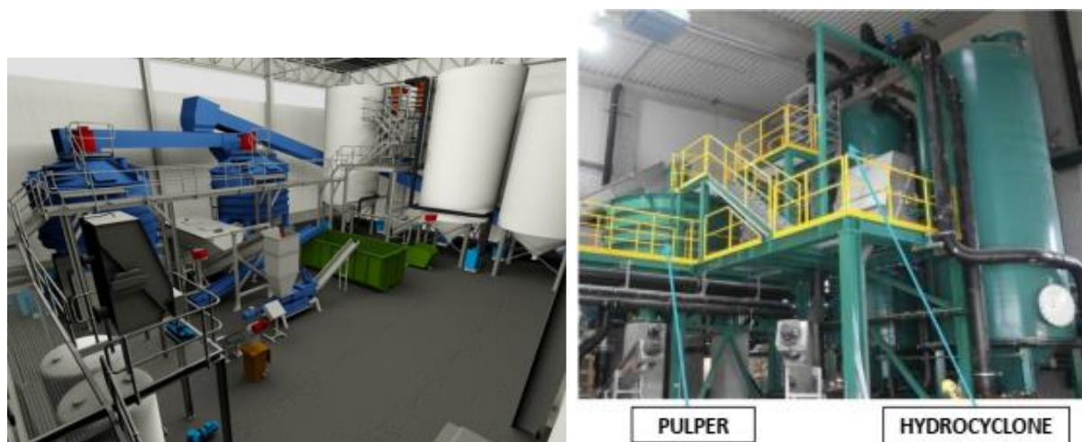
Figură 3-63 Sistemul pulper și hidrociclon
