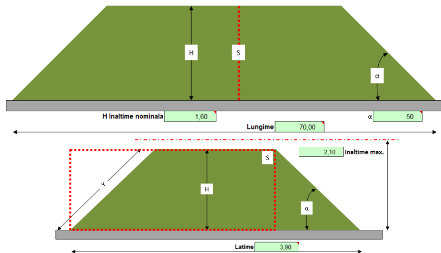
Figură 3-45 SC Șura Mică – maturare: Dimensiuni a brazdelor de maturare
