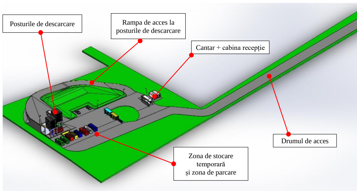
Figură 3-25 Stația de Transfer Avrighi – perspectivă
