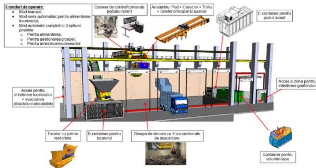
Figură 3-49 TMB cu bioscări – exemplu recepție groapă cu pod rulant și graifer
