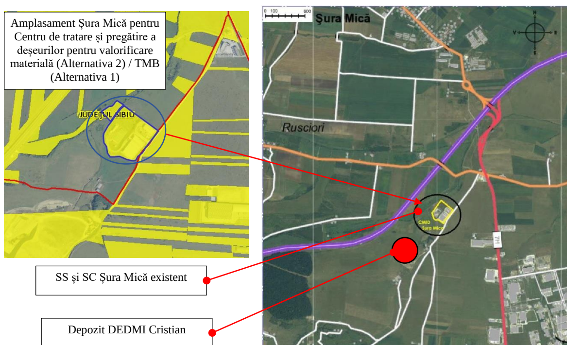
Figură 3-17 Instalație de Digestie Anaerobă / TMB - Plan amplasament propus
