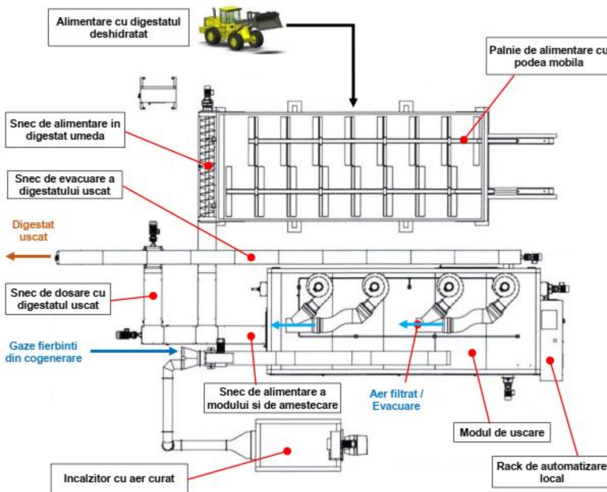
Figură 3-73 – Principiu de funcționare al unei unități de uscare cu 1 modul de uscare
