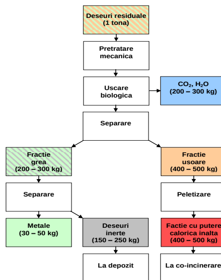
Figură 3-9 – TMB cu biousoare – schemă flux
