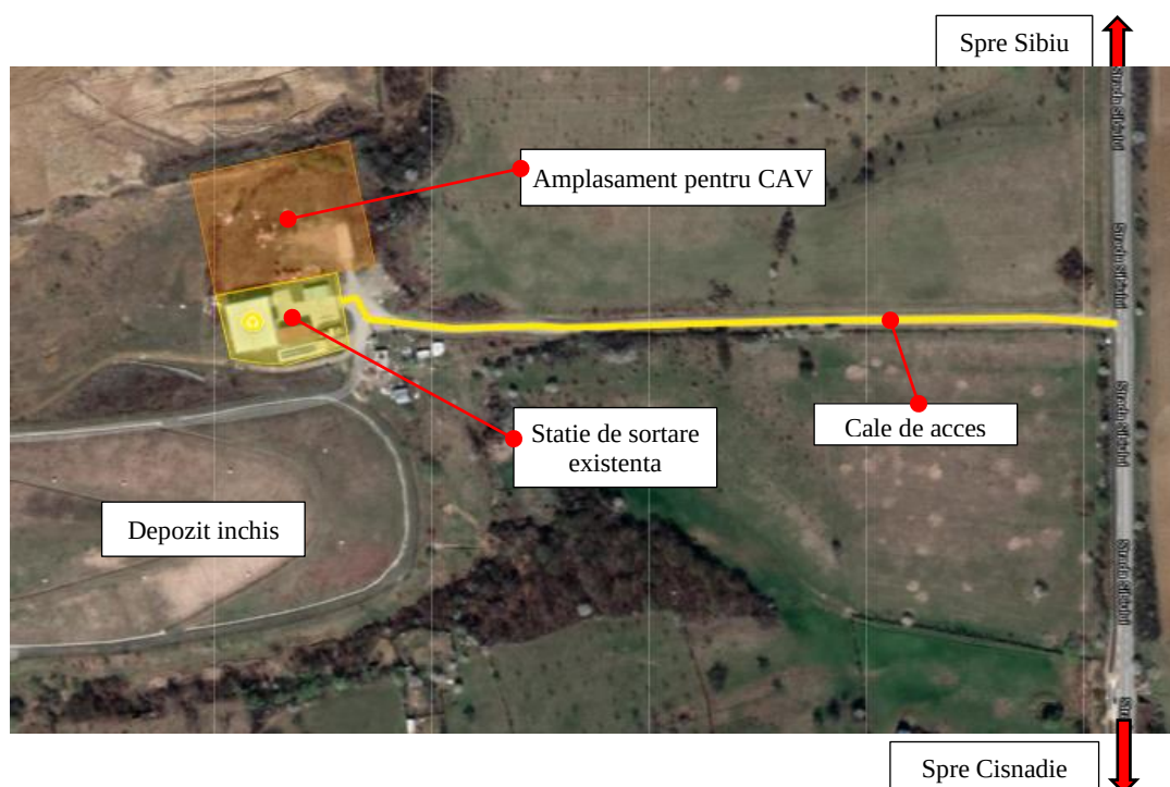
Figură 3-28 CAV Cisnădie – plan amplasament
