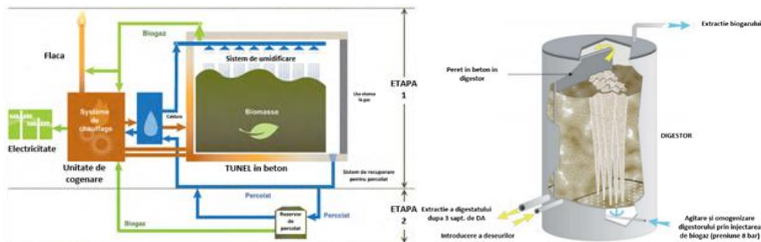
Figură 3-6 – Digestie anaerobă uscată (exemplu)
