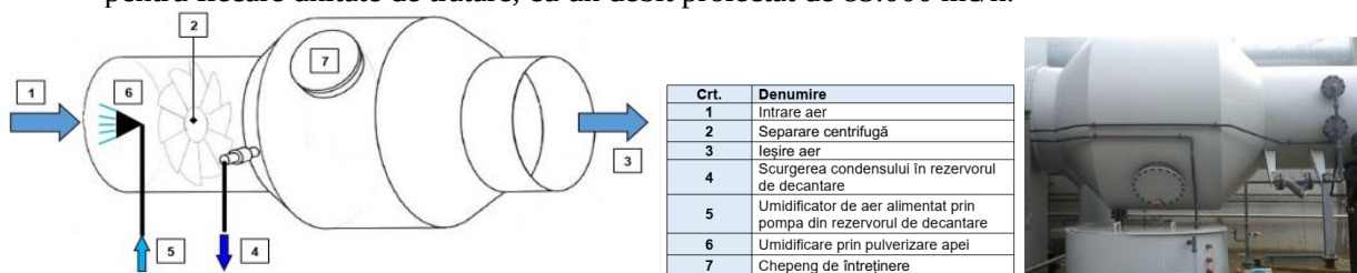
Figură 3-75 Sistem de desprăfuire - principiu de funcționare și exemplu
