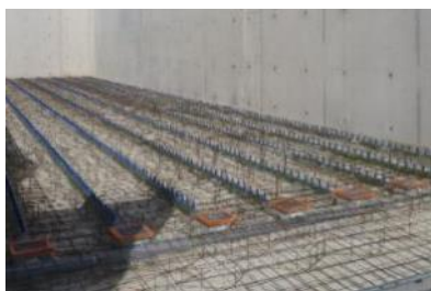
Figură 3-44 SC Sura Mica – exemple: conducte aerare; sistem umidificare; sistem aspirație aer
