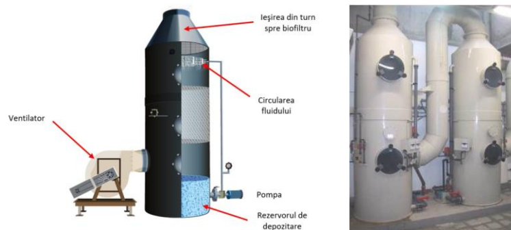
Figură 3-76 Sistemul de epurare (scrubber acid) – principiu de funcționare și exemplu
