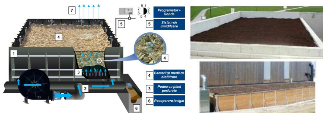
Figură 3-77 Biofiltru – principiu de funcționare și exemplu
