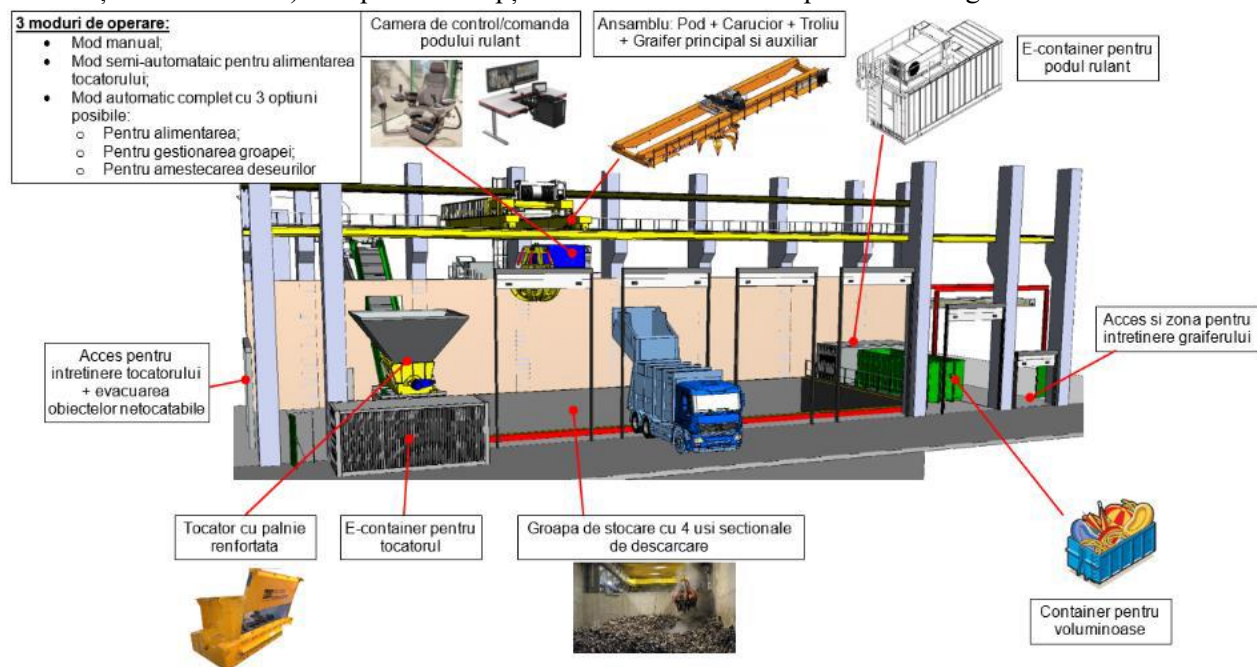
Figură 3-56 Principiul de funcționare al modului de recepție cu groapă și pod rulant cu greifer
