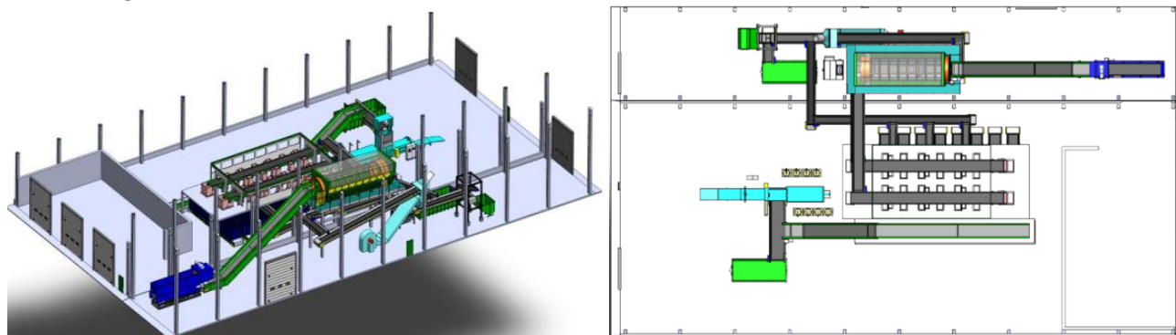
Figură 3-52 Perspectivă și vedere de sus a liniei de sortare hârtie/carton propuse
