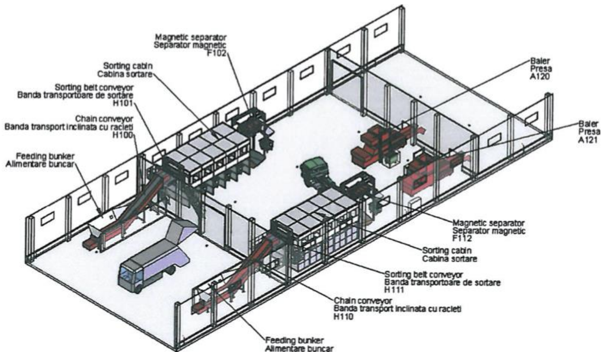
Figură 2-22 – Schema Stație de Sortare Șura Mică
