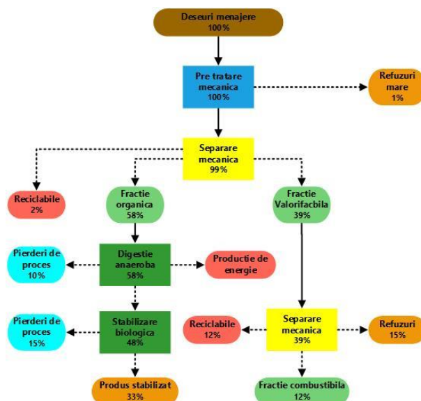
Figură 3-10 – TMB cu digestie anaerobă – schemă flux
