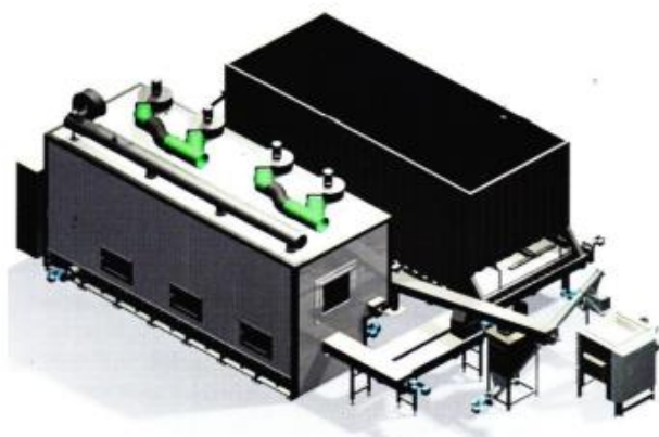
Figură 3-72 Exemplu de unitate de uscare
