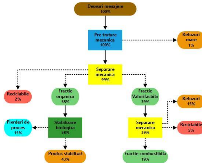
Figură 3-8 – TMB cu bio-stabilizare – schemă flux
