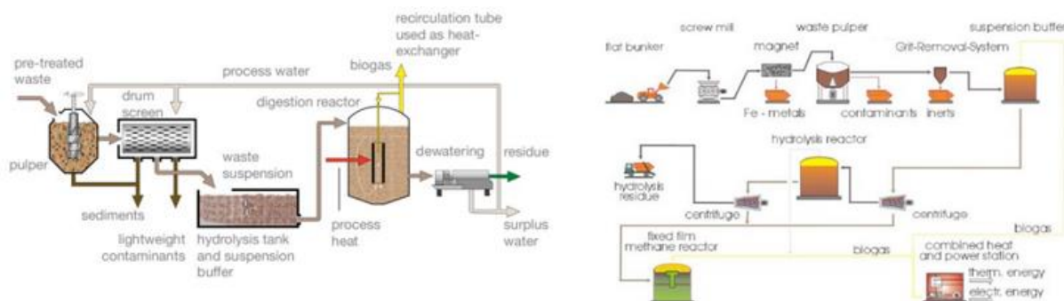
Figură 3-5 – Digestie anaerobă umedă (exemplu)
