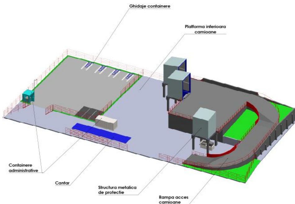
Figură 3-26 Stația de Transfer Agnita – perspectivă
