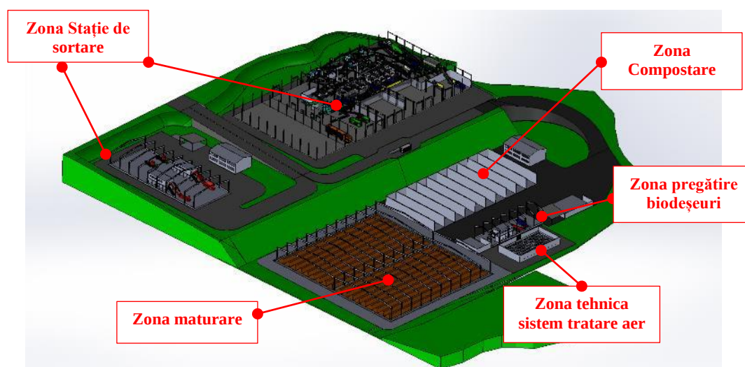
Figură 3-40 SC Sura Mica – plan de situație
