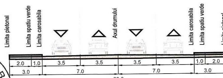
Profil transversal propus A-A' sc:1/200 Drumul Agatului
