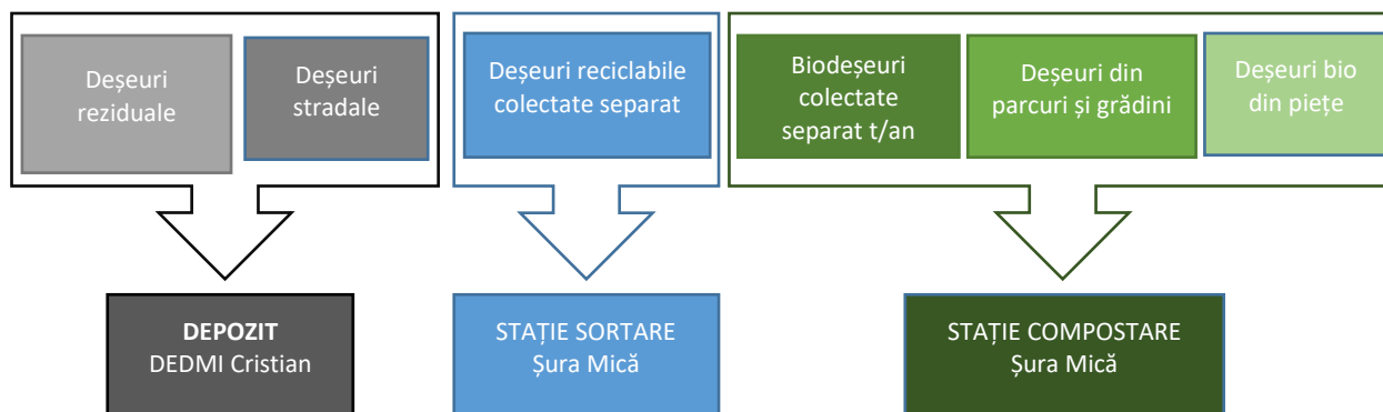
Figură 2-6 Zona 1 – Sibiu - Flux deșeuri
