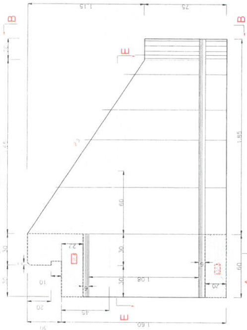
SECȚIUNE C-C Sc. 1:25
